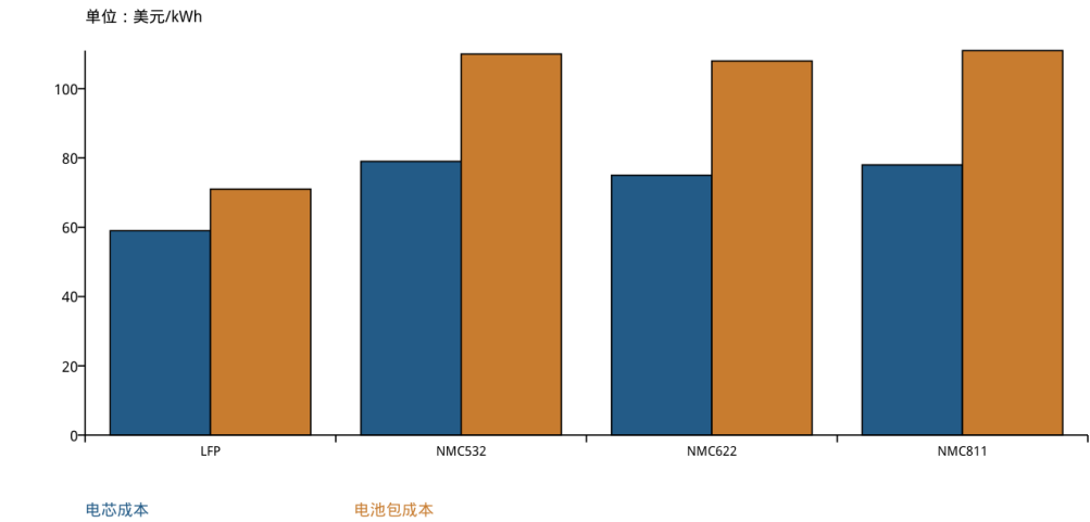
电池电芯与电池包现货成本
