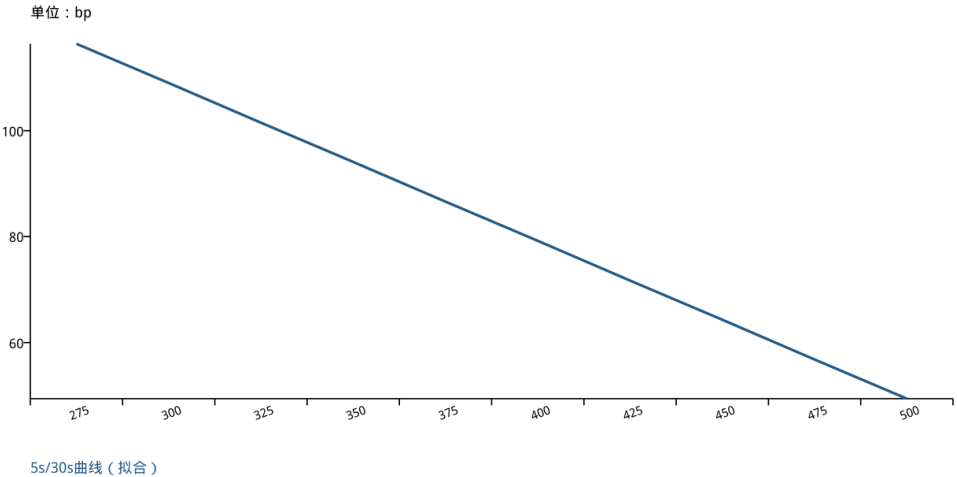
5s/30s美债曲线对1y1y OIS的回归（近一年，单位：bp）
