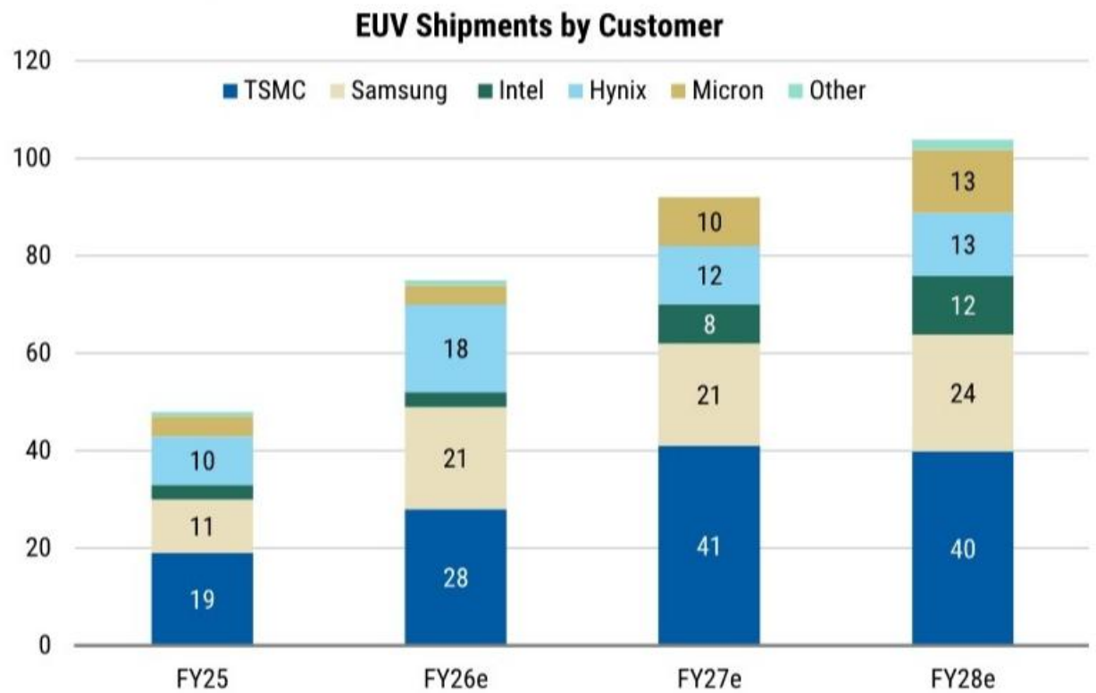
图表2：我们预计2027财年和2028财年EUV出货量分别为92台和104台。
