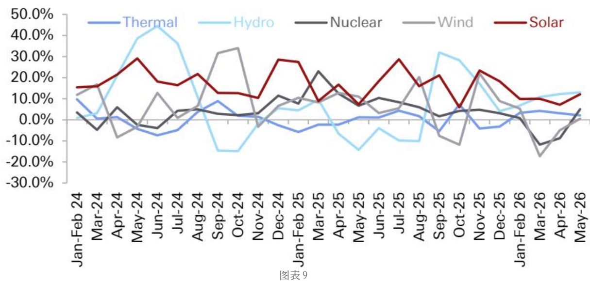
图9：中国 – 按燃料类型划分的月度发电量（同比）
