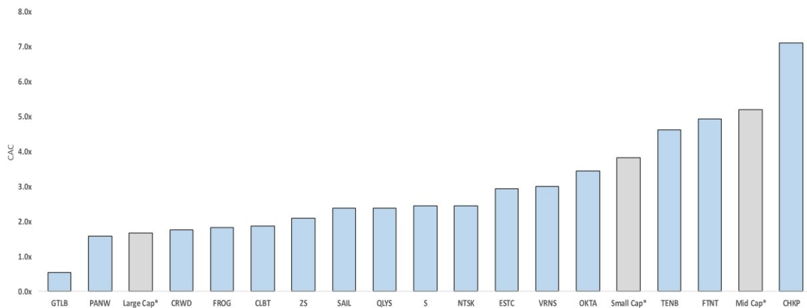
CAC
