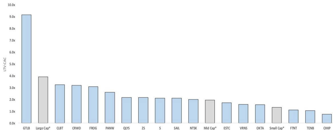
LTV:CAC
