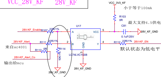
KF驱动器 28V供电控制电路
