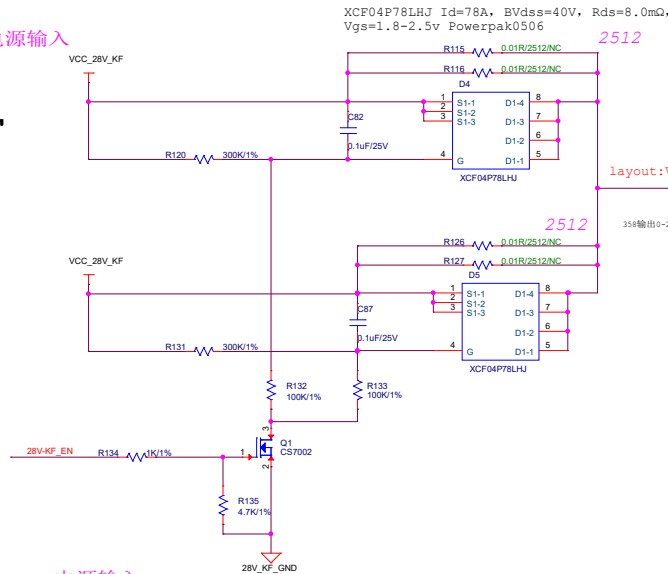
电源输入
