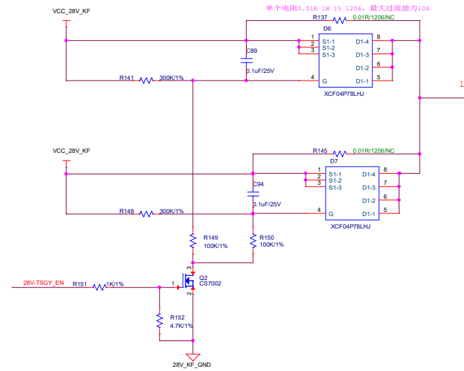
电源输入
