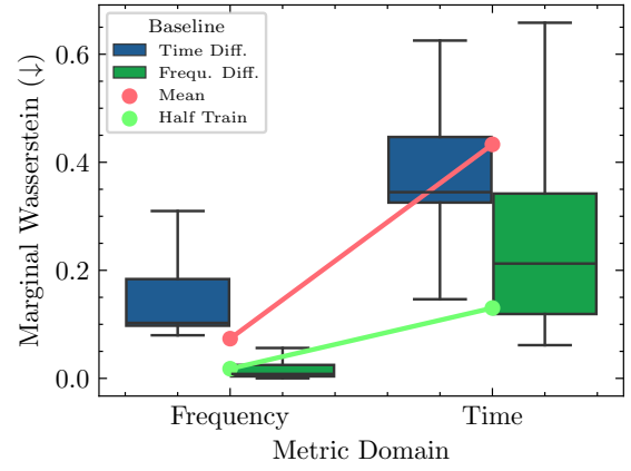
(d) NASA-Charge.
