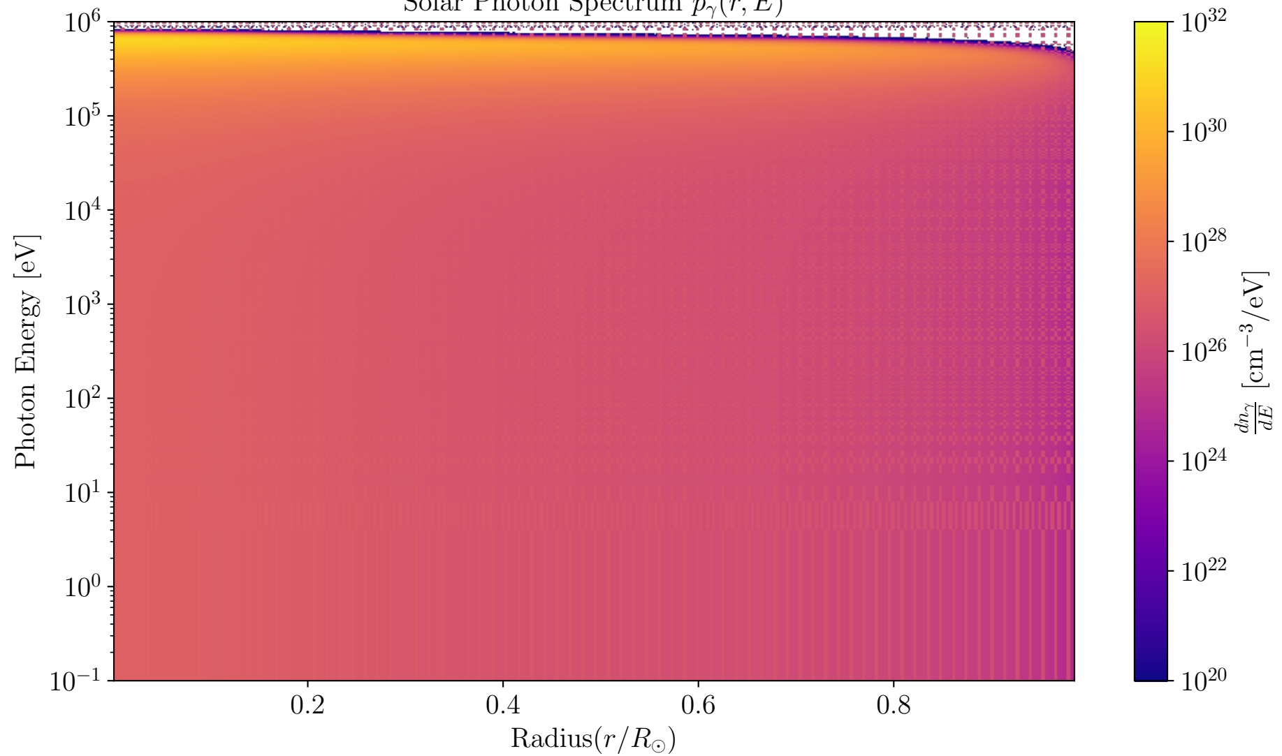
Solar Photon Spectrum p_\gamma(r, E)
