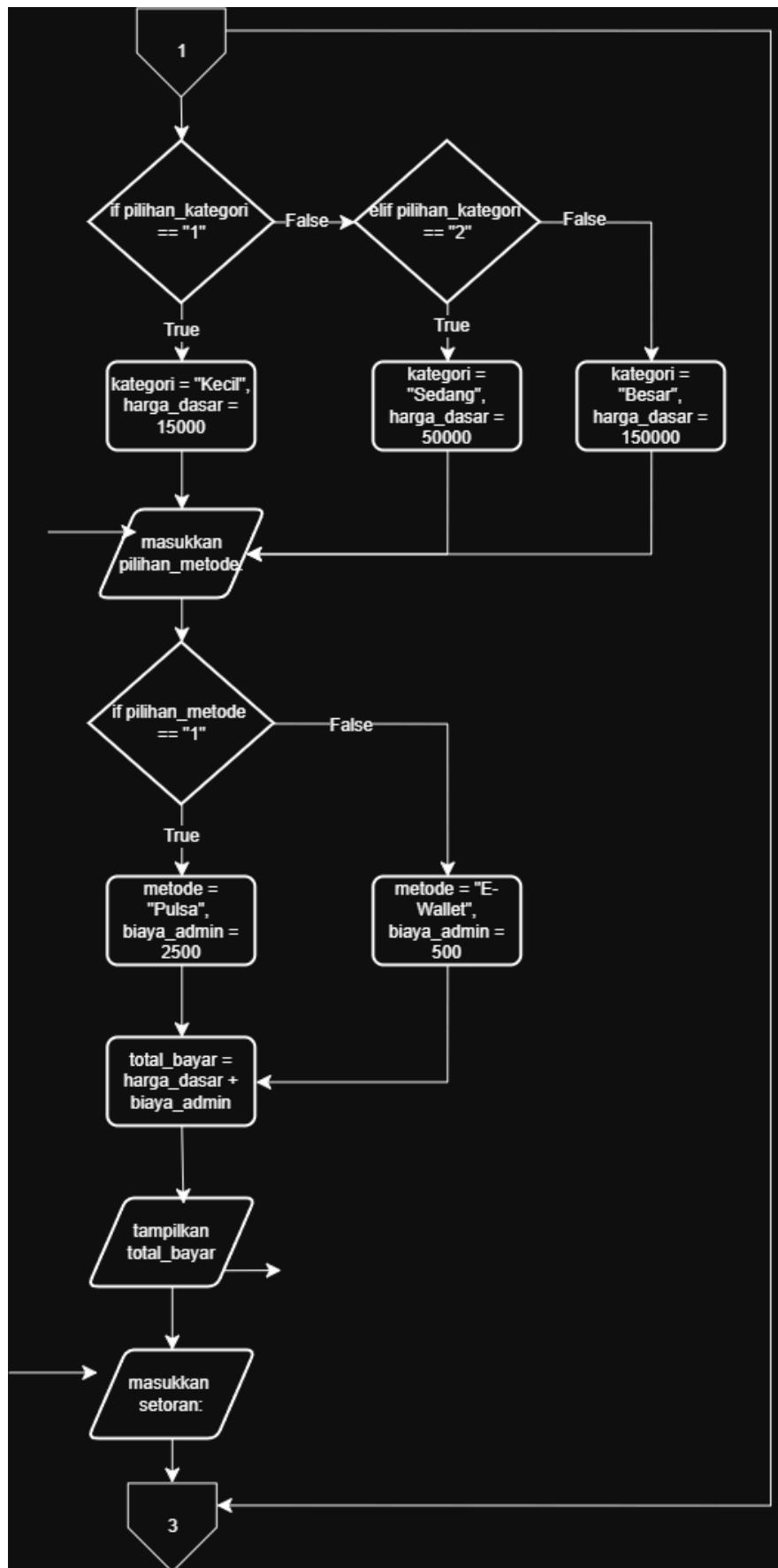
Gambar 1.2 Flowchart di Halaman ke-2
