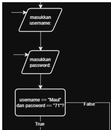
Gambar 1.4 Validasi Login di Halaman ke-1
