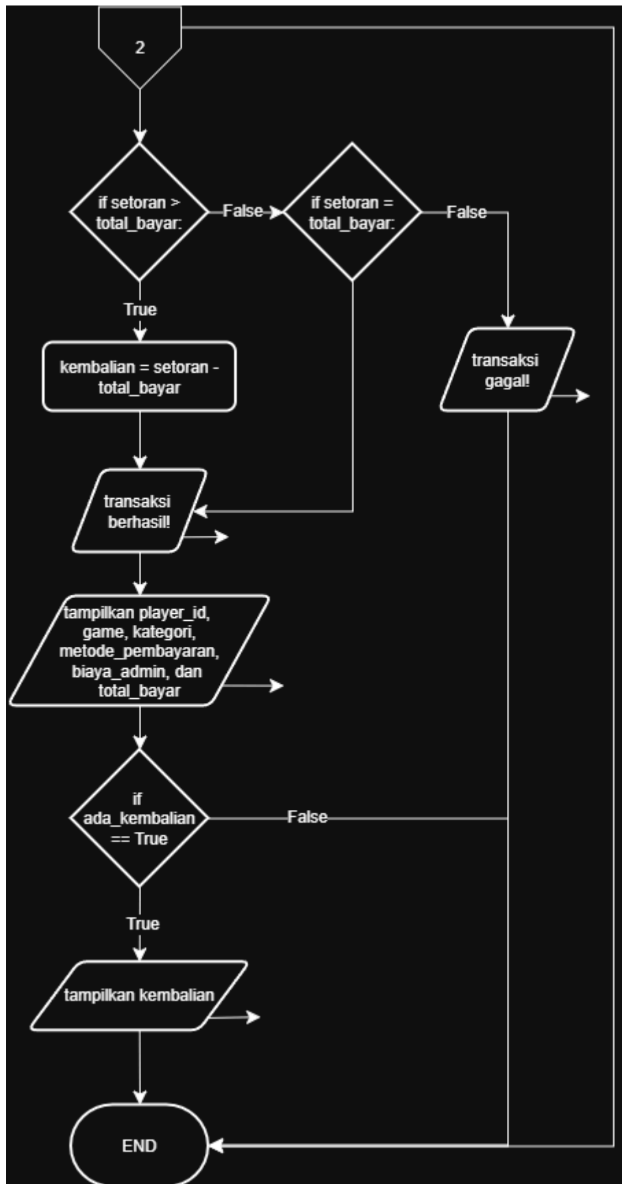
Gambar 1.3 Flowchart di Halaman ke-3
