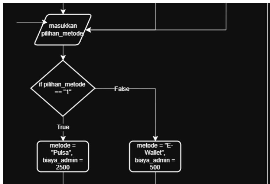
Gambar 1.7 Assign metode dan biaya_admin berdasarkan pilihan_metode
