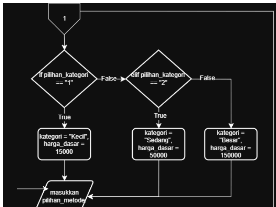
Gambar 1.6 Assign kategori dan harga_dasar
