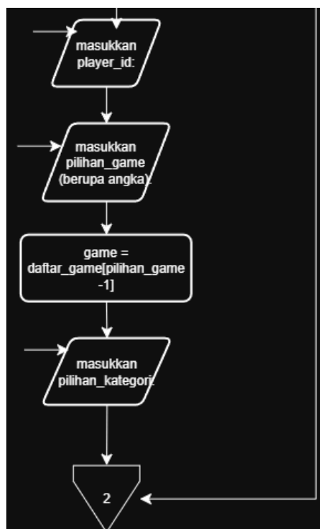
Gambar 1.5 Permintaan Memasukkan player_id , pilihan game , dan pilihan kategori
