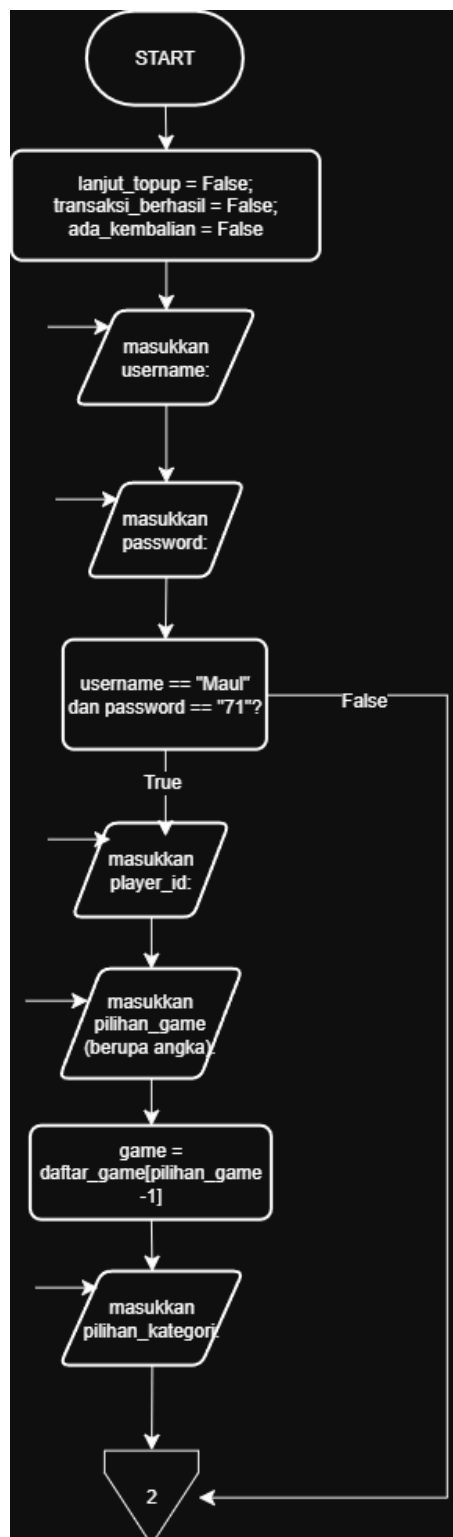
Gambar 1.1 Flowchart di Halaman ke-1
