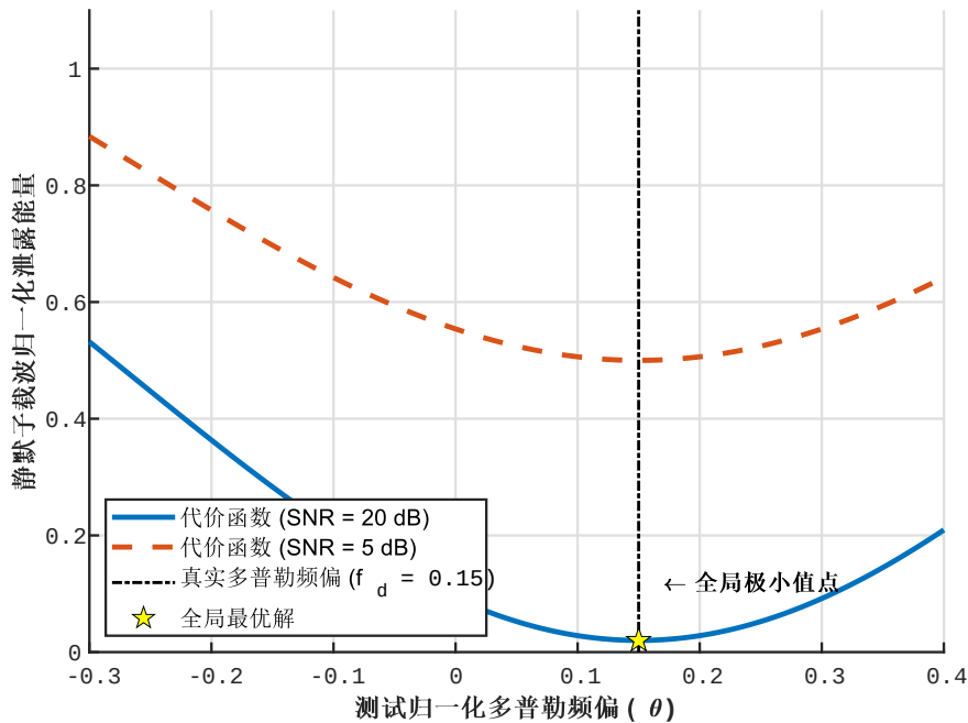
图 4.4 静默位置泄露能量代价函数随试探频偏参数的变化曲线
