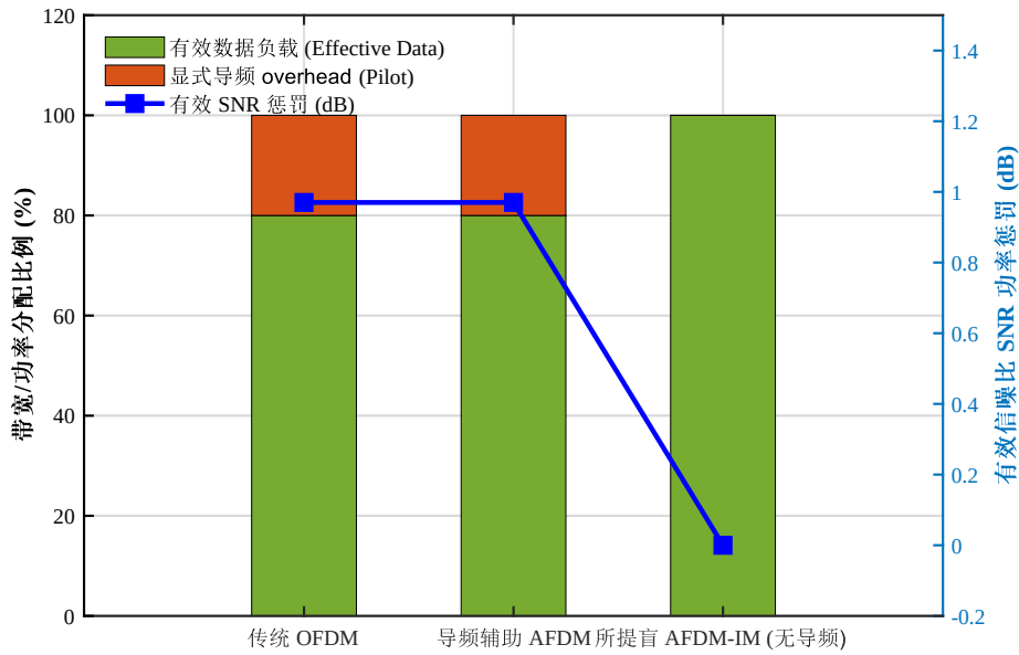
图 4.8 不同方案的资源分配对比与导频开销引起的等效 SNR 惩罚
