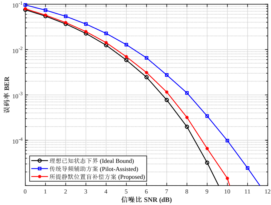
图 4.7 不同残余 CFO 补偿策略下相干 AFDM-IM 系统的 BER 性能对比
