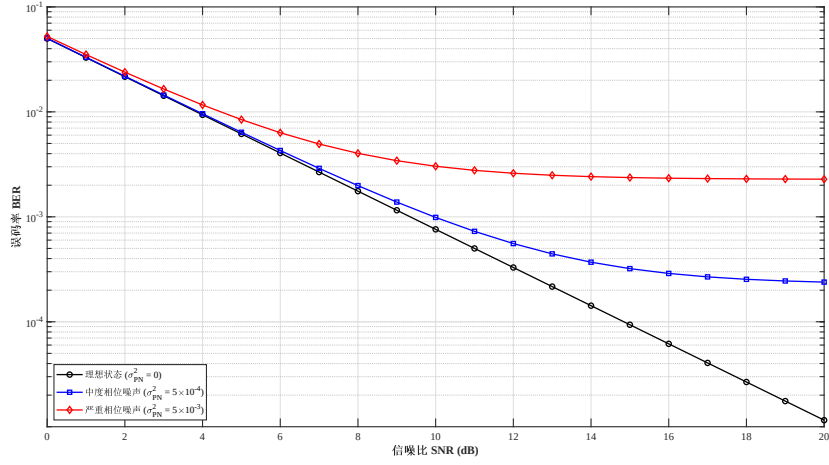
图 4.9 不同激光器线宽条件下相干 AFDM-IM 系统的 BER 性能
