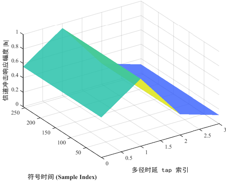
图 4.5 高动态水下信道冲激响应三维演化图 ( N = 256 , P = 4 , f_d = 0.15 )
