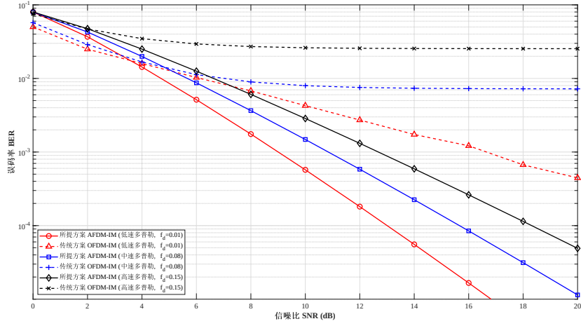
图 4.6 高动态场景下不同相干索引调制方案的 BER 性能对比
