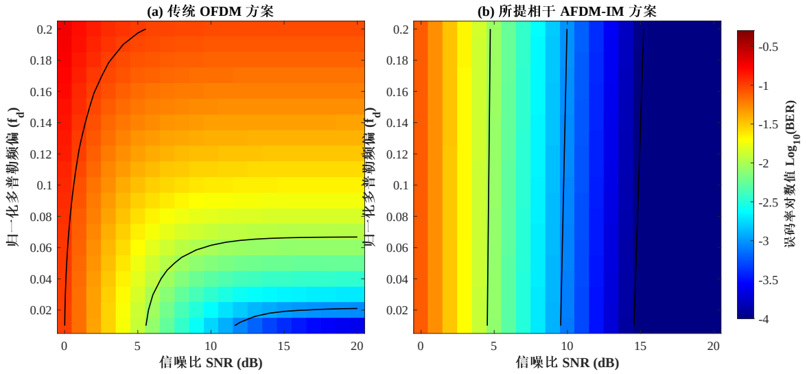
图 4.10 不同归一化多普勒频移与 SNR 条件下的 BER 二维热力图对比
