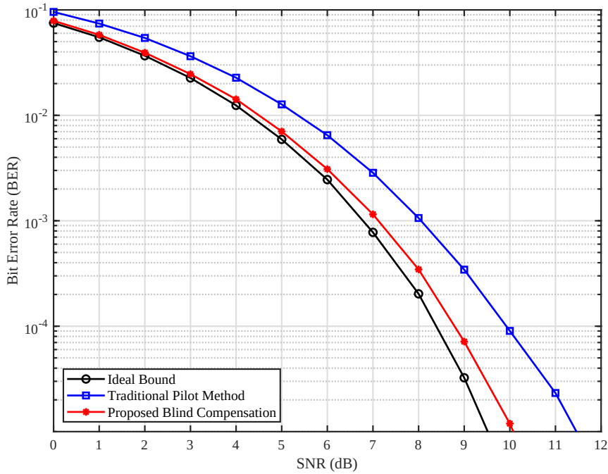
图 4.3 不同残余 CFO 补偿策略下相干 AFDM-IM 系统的 BER 性能对比
