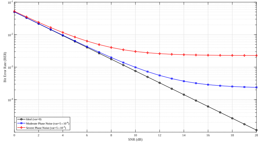
图 4.4 不同激光器线宽条件下相干 AFDM-IM 系统的 BER 性能
