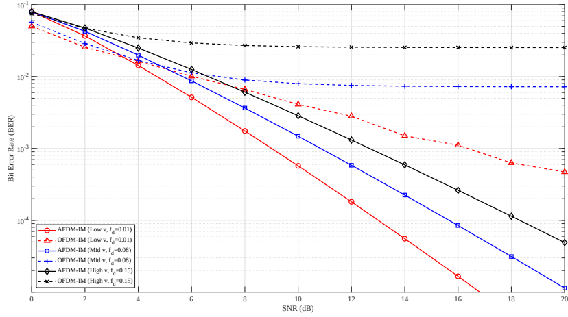
图 4.2 高动态场景下不同相干索引调制方案的 BER 性能对比
