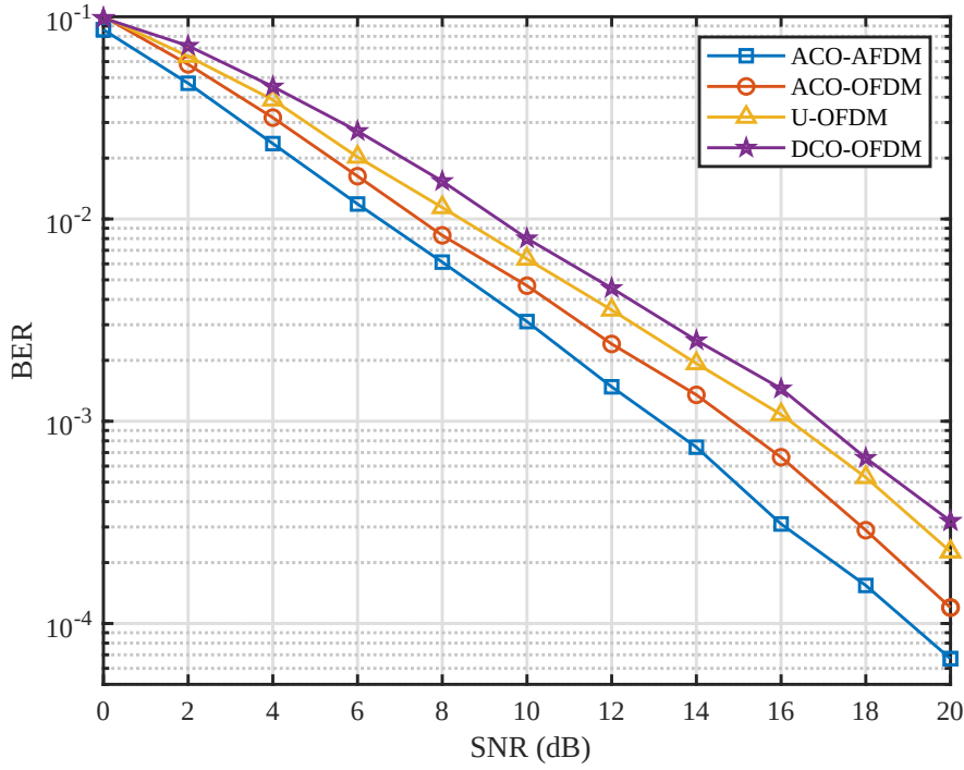
图 3.2 不同多载波方案在两径信道下的误码率性能对比
