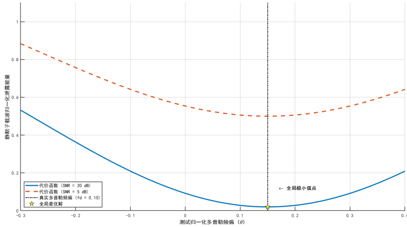
图 4.3 静默位置泄露能量代价函数随试探频偏参数的变化曲线
