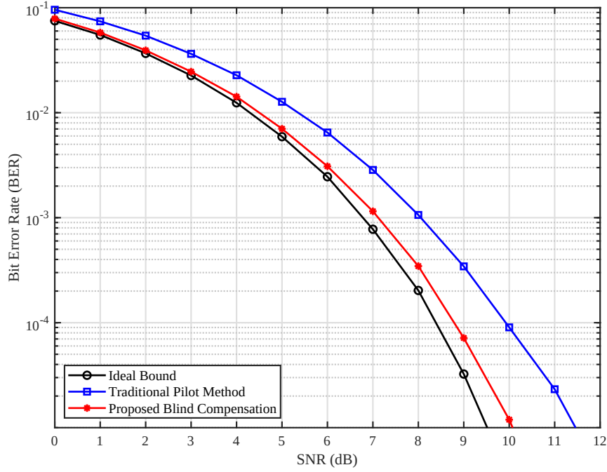
图 4.6 不同残余 CFO 补偿策略下相干 AFDM-IM 系统的 BER 性能对比
