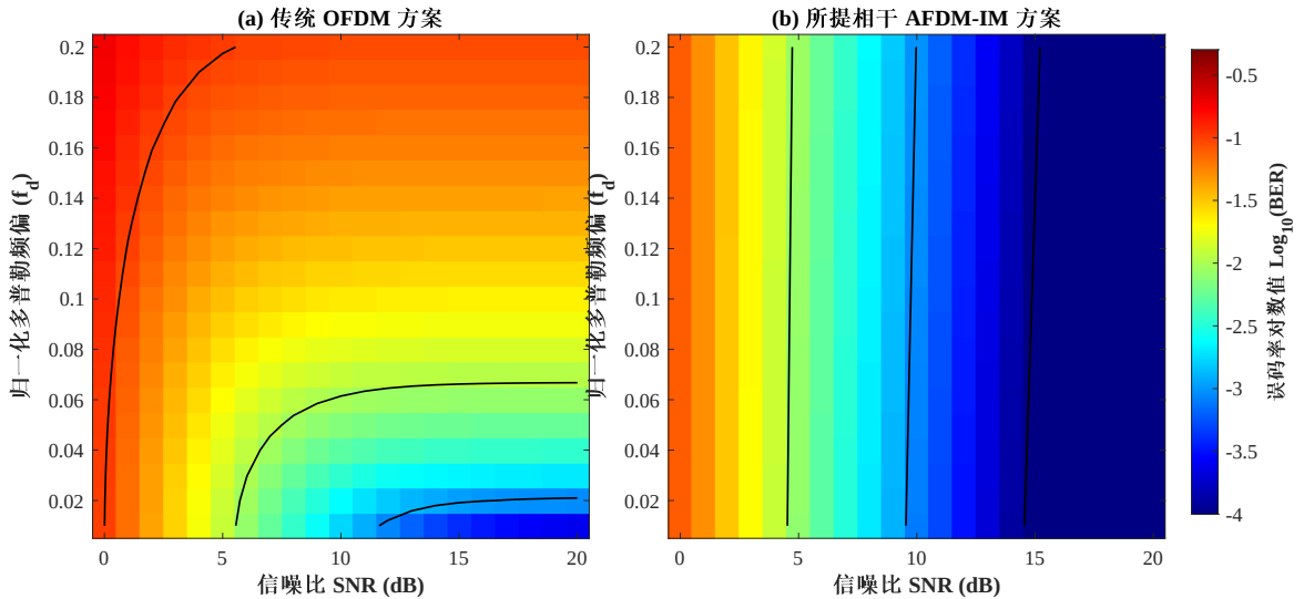
图 4.9 不同归一化多普勒频移与 SNR 条件下的 BER 二维热力图对比
