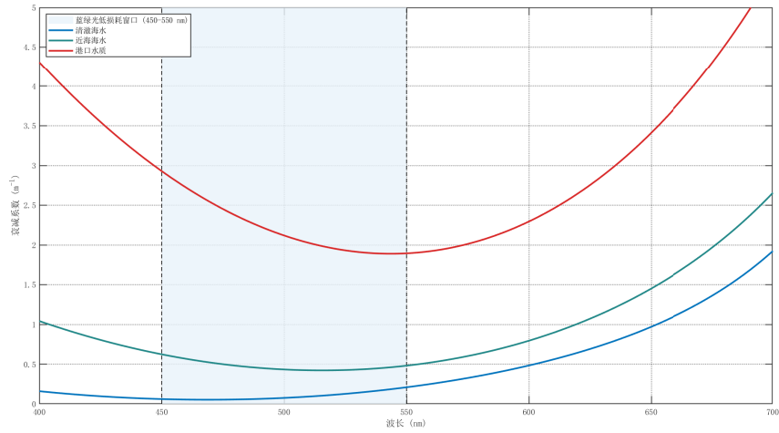
图 2.1 不同水质条件下光衰减系数随波长变化曲线
