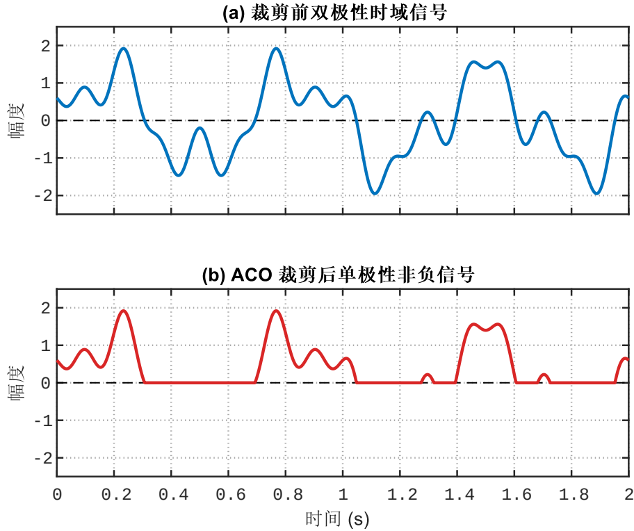
图 3.2 ACO 非对称限幅下的单极性非负时域波形变换示意图
