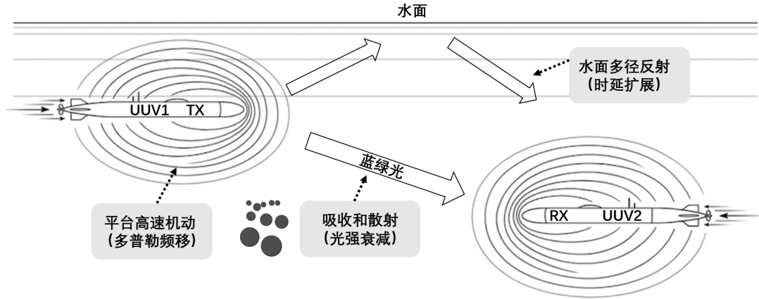
图 1.1 水下无线光通信典型应用场景及主要信道挑战示意图
