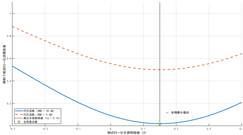
图 4.6 静默位置泄露能量代价函数随试探频偏参数的变化曲线
