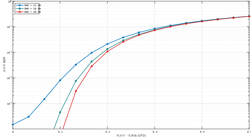
图 4.4 不同残余 CFO 失配程度下相干 AFDM-IM 系统的 BER 敏感性曲线
