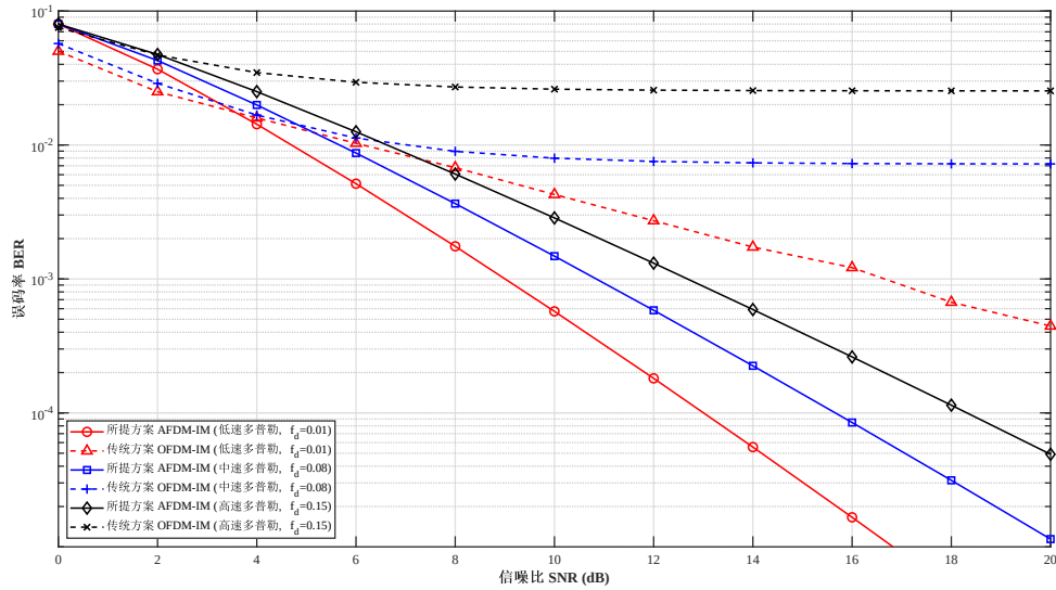
图 4.8 高动态场景下不同相干索引调制方案的 BER 性能对比
