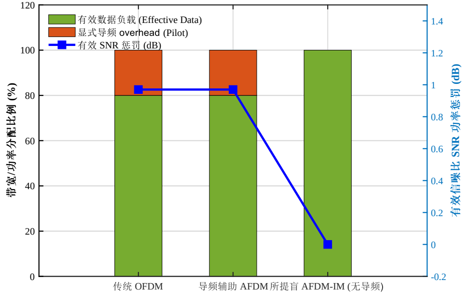
图 4.10 不同方案的资源分配对比与导频开销引起的等效 SNR 惩罚
