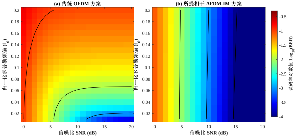
图 4.12 不同归一化多普勒频移与 SNR 条件下的 BER 二维热力图对比
