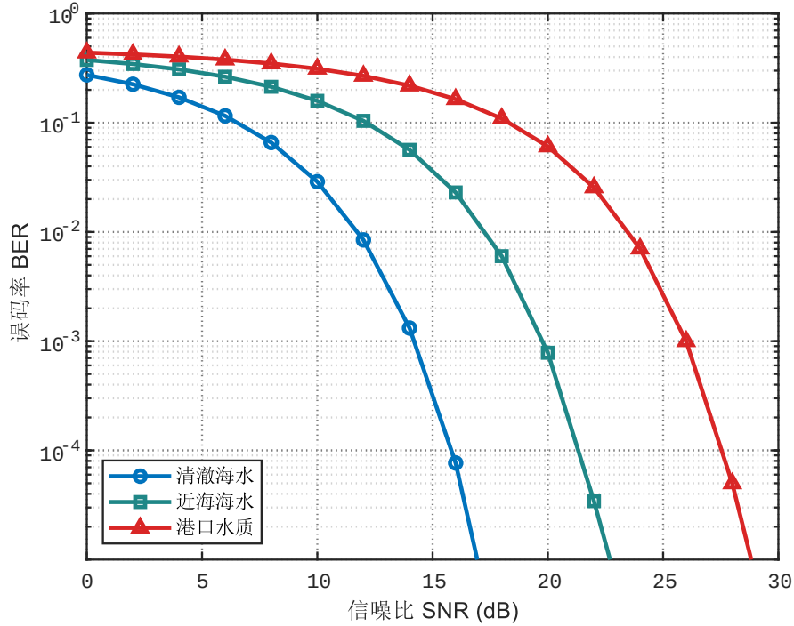
图 3.5 不同水体环境下 ACO-AFDM 系统的 BER 性能对比
