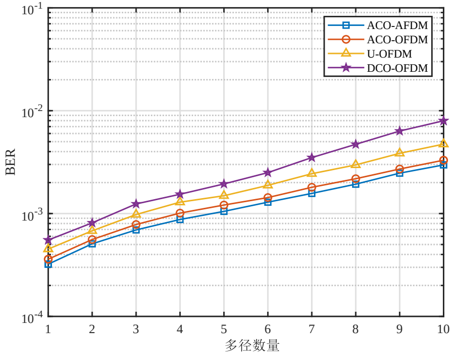
图 3.4 多径路径数量对系统误码率性能的影响
