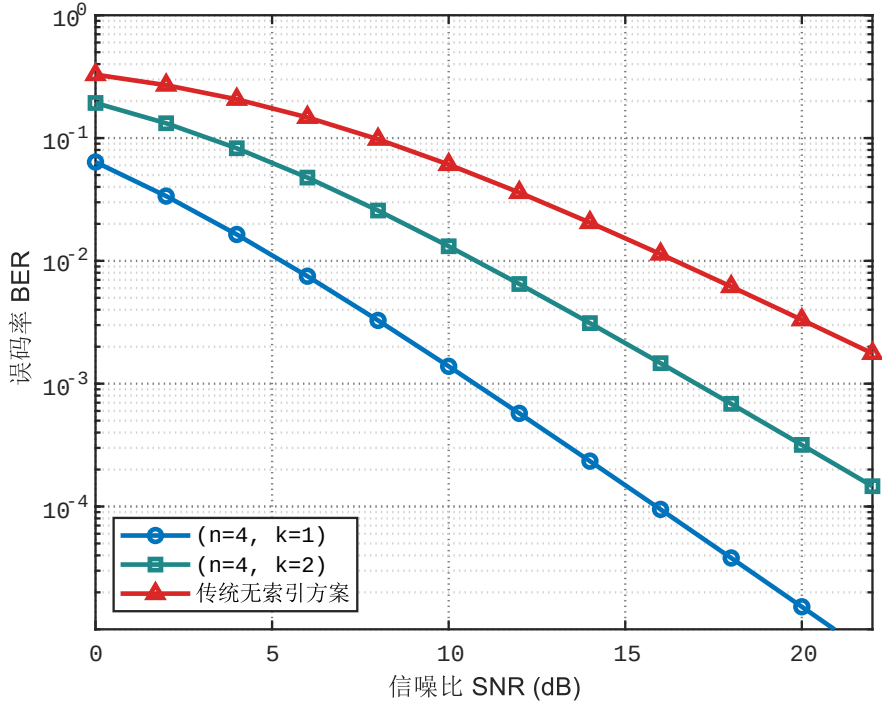
图 4.3 不同子块映射模式 (n, k) 下相干 AFDM-IM 系统的 BER 性能对比 发送向量经离散逆傅里叶变换映射至时域。记 AFDM 调制矩阵为
