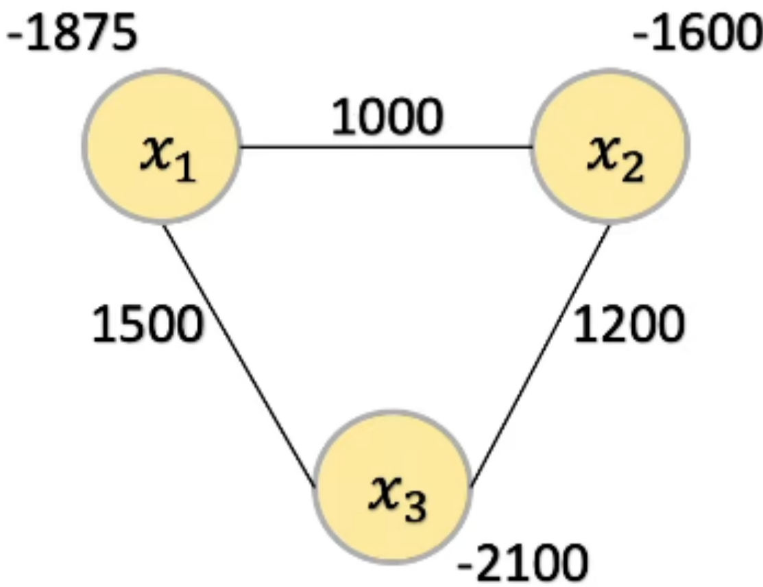
QUBO
