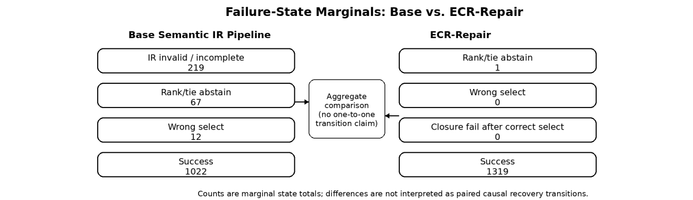
Figure 3: Base Semantic IR Pipeline 与 ECR-REPAIR 的失败状态压缩概览。该图用于展示边际失败量级变化，不将总量差直接解释为逐样本因果转移。
