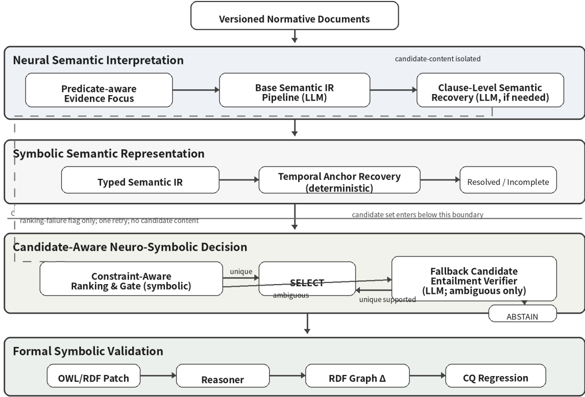
Figure 1: ECR-REPAIR的证据约束神经符号总体架构。 Semantic IR 是神经到符号语义接口；候选集合仅在候选感知决策层可见。 Fallback Candidate Entailment Verifier 只在符号排序存在歧义时触发，虚线反馈只携带不含候选语义的排序失败标志。
