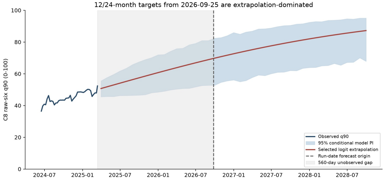
图 15 有界 logit 前沿的条件预测扇形。统计区间未包含模型选择 来源误差及缺失训练量的不确定性，两期限均为长期外推。
