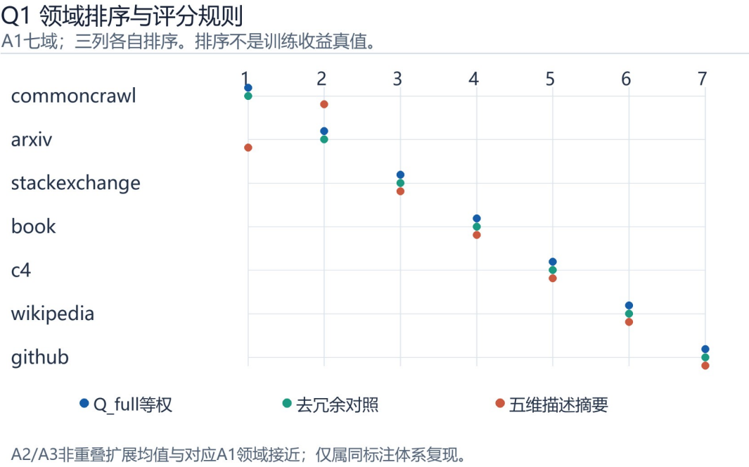
图 3 A1 七域的 Q_full 等权、去冗余 W1 与五维 DQ0 独立排序。A2、A3 非重叠扩展均值与对应领域接近；这些均属标注体系内的描述结果。
