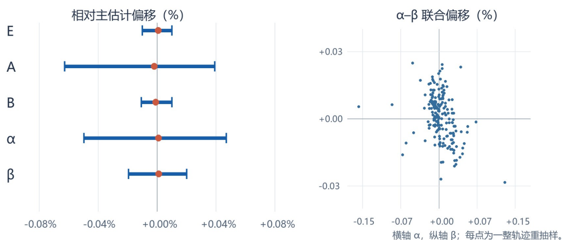
图9 二百次整轨迹重抽样的五参数相对主估计条件分位及 \alpha — \beta 联合散点。每点为一次整轨迹重抽样，区间不覆盖来源和模型错误。
