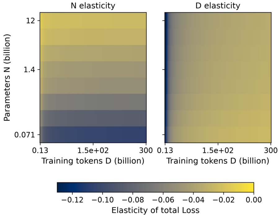
图 6 参数与数据规模对总 Loss 的弹性热图。横纵轴按 B1 网格位置排布；图中没有有限替代曲线，替代关系由式（9）给出。
