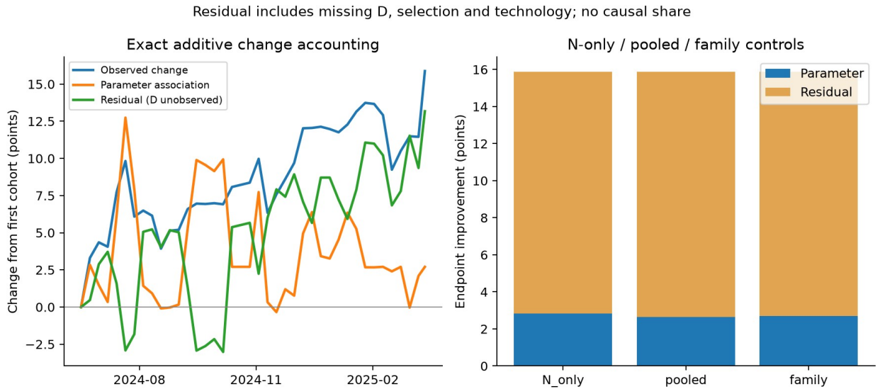
图 14 前沿变化的参数关联与调整残差分解。两分量相加等于前沿，不表示完整规模与因果技术贡献。
