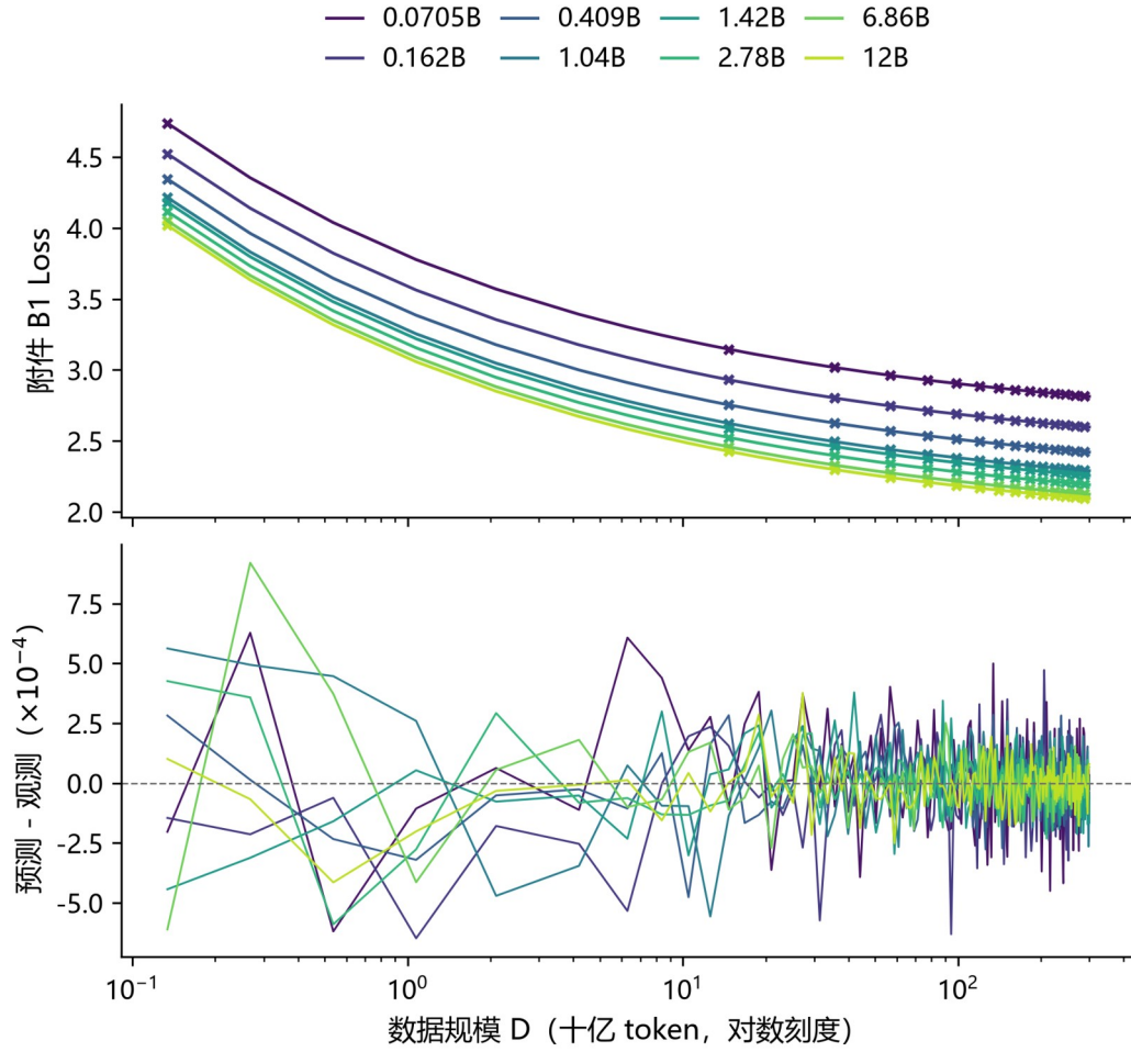
图 7 B1 八条完整训练轨迹的观测、拟合与残差。检查点之间相关；图形只核验当前附件内部的加性幂律形状。
