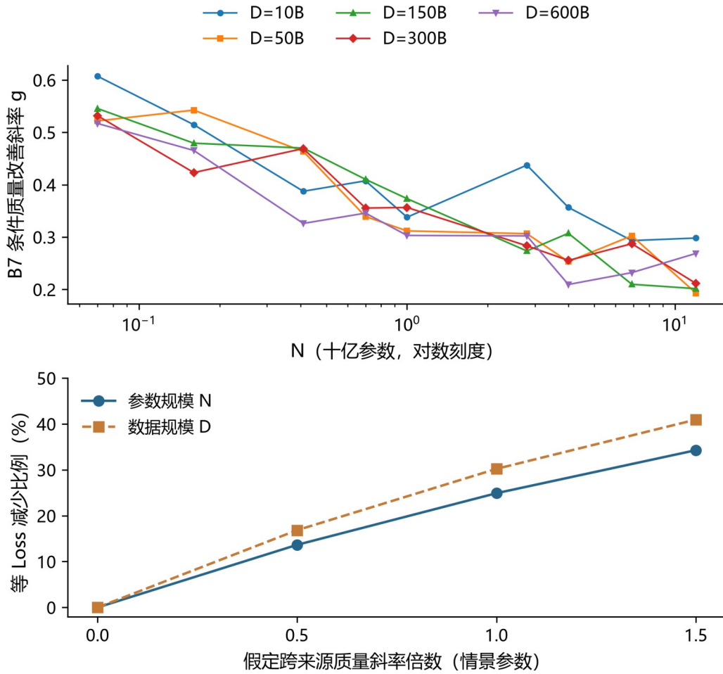
图 10 B7 半合成单元的质量改善斜率及假定质量运输下的有限替代。上图是半合成表内形状，下图是条件情景，不是观测训练回报。
