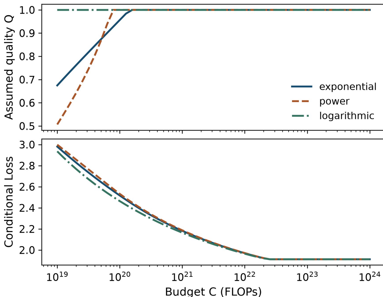
图 12 三种题设质量成本下的条件 Q 与 Loss 路径。收益假设来自半合成质量校准，曲线不是实测投资回报。
