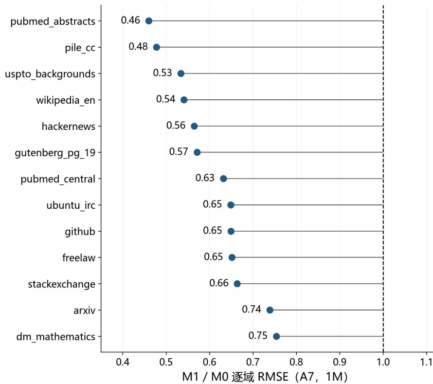
图 4 1M 留出样本的逐领域预测误差。全 13 域改善仍伴随不同的误差水平，完整数值见附录 B。
