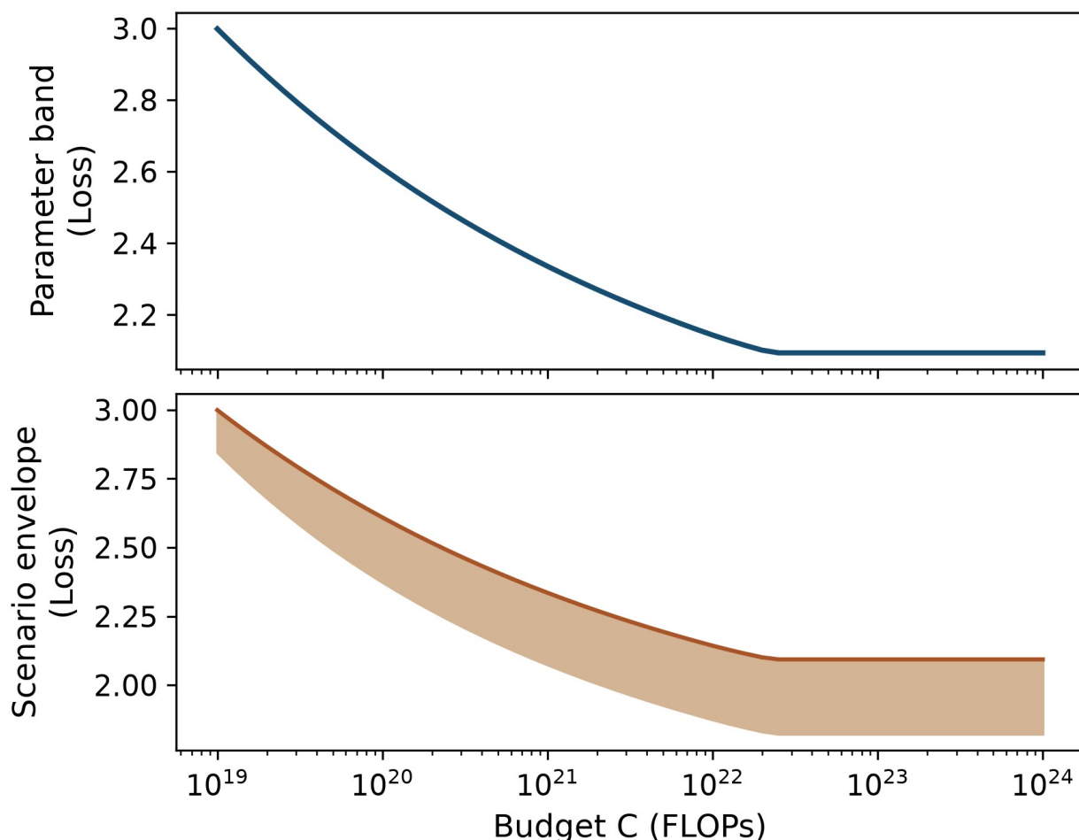
图 13 联合参数传播与机制情景范围。上图为条件参数带，下图为不同成本与收益机制的情景包络，后者不是置信区间。
