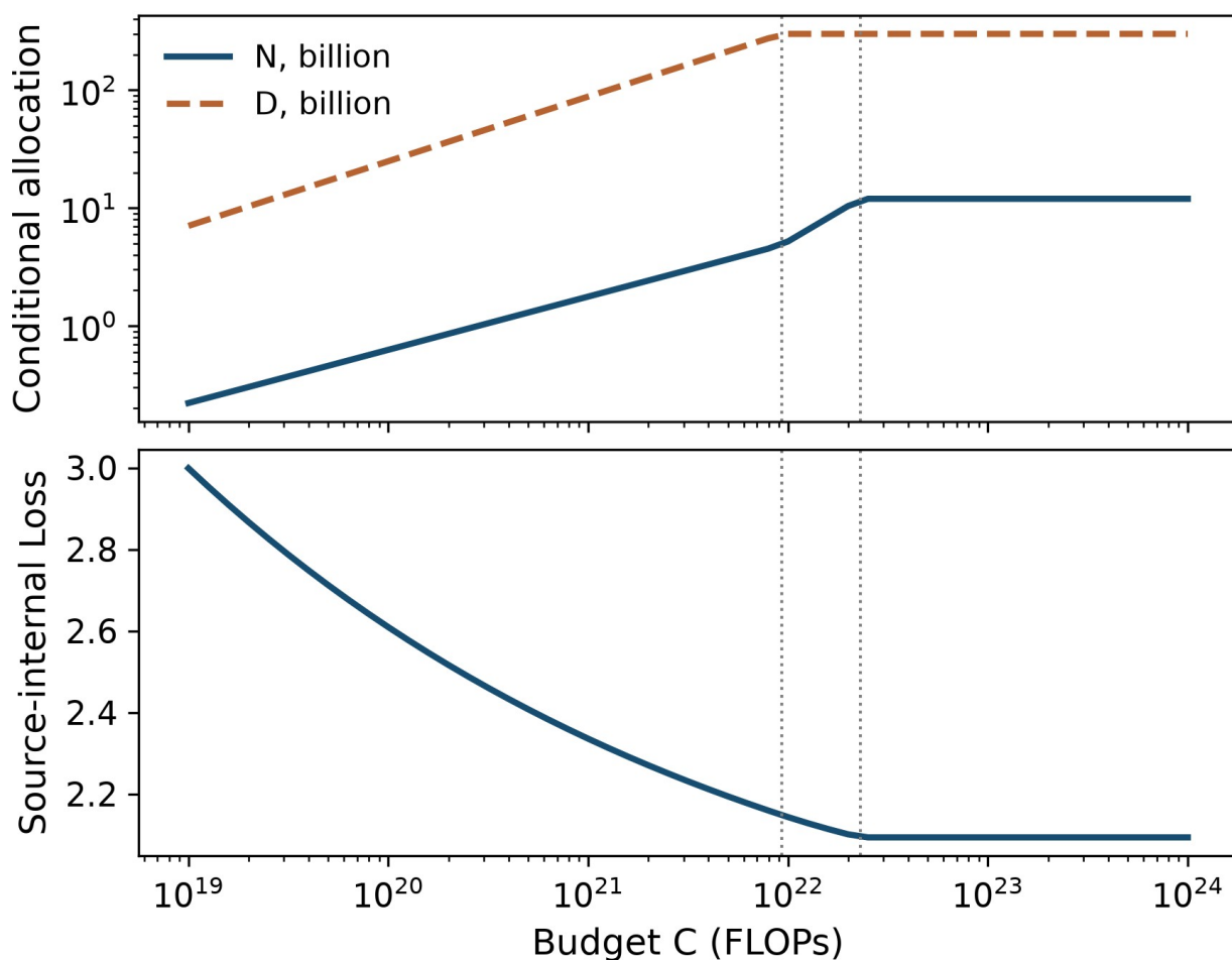
图 11 题设成本代理与附件内部 Loss 下的预算配置及损失路径。竖向点线标示统计支持界开始活跃的位置；橙色虚线为最优数据量，平台不代表真实训练收益终极饱和。
