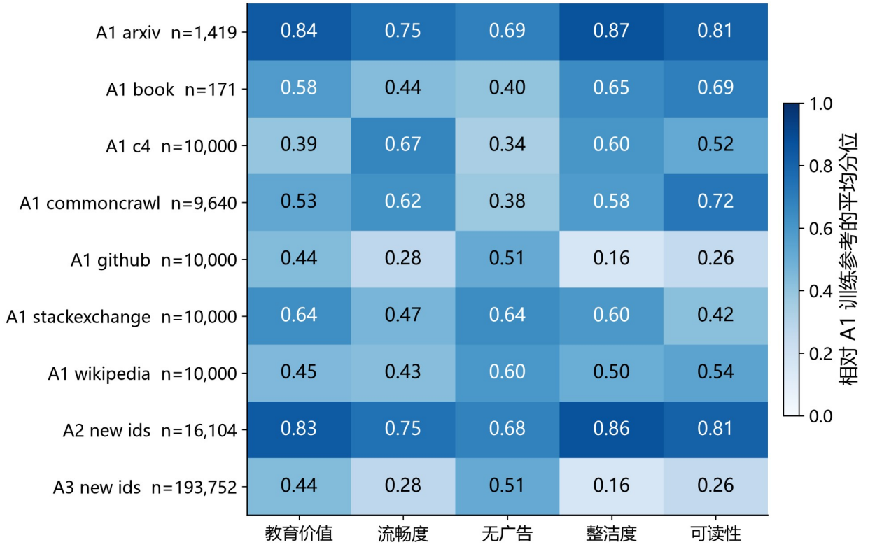
图 2 五维质量在抽样及扩展领域中的描述画像。横向比较依赖相同参考分布，不能解释为真实训练收益排序。
