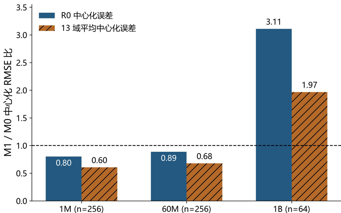
图 5 冻结 M1 相对于 M0 的跨规模中心化误差比。1M 有局部留出收益，60M 仅部分迁移，1B 失败；10B、70B 估算表另作压力检查。
