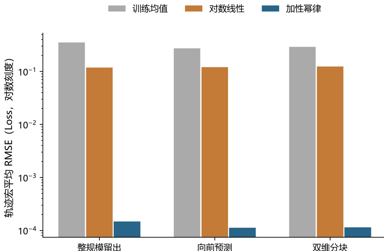
图 8 幂律模型与两类基准的分组验证。纵轴量尺和对数刻度见原图；极小误差只对应本附件内部。
