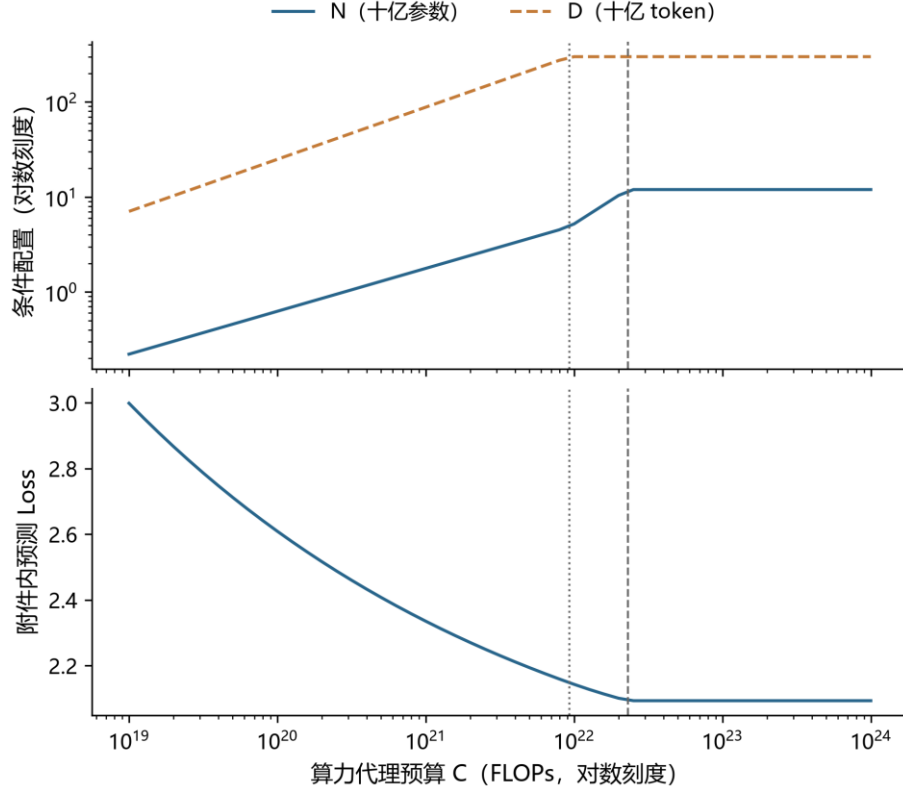
图 5 参考上下文下的预算配置及 Loss 路径。高预算平台反映统计支持上限，非真实训练收益终极饱和。
