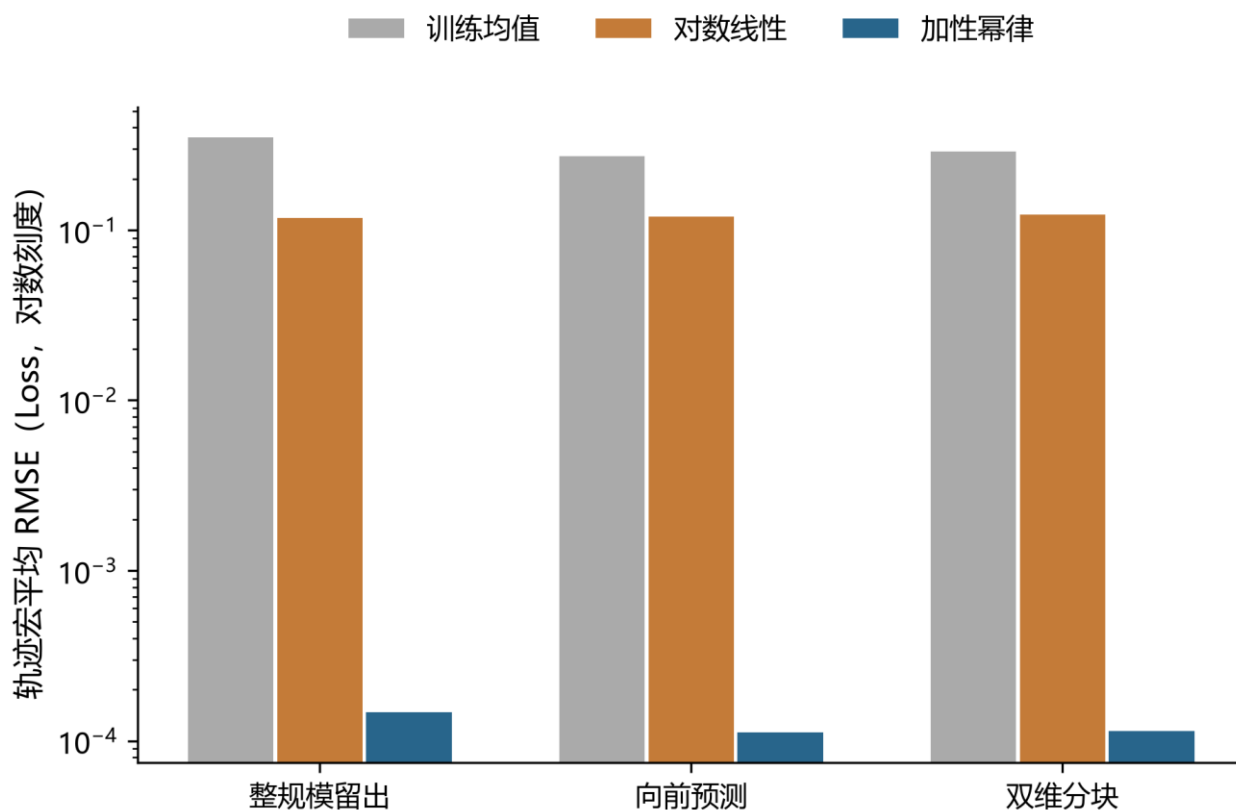
图 3 幂律模型与两类基准的分组验证。纵轴量尺和对数刻度见原图；极小误差只对应本附件内部。
