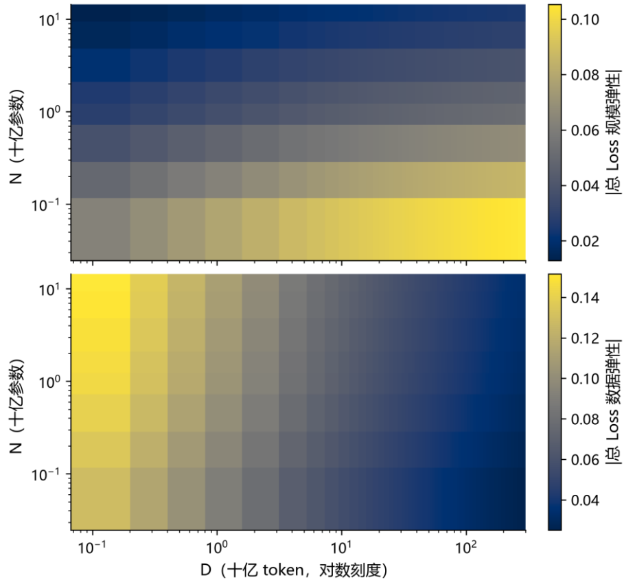
图 4 参数 数据的边际与替代关系。所有数量采用十亿单位；示例局部导数不能直接外推为有限变化。
