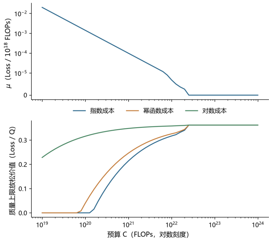
图 11 条件预算影子价格路径。支持上界同时活跃后乘子为零，仅对应给定目标与统计支持约束。
