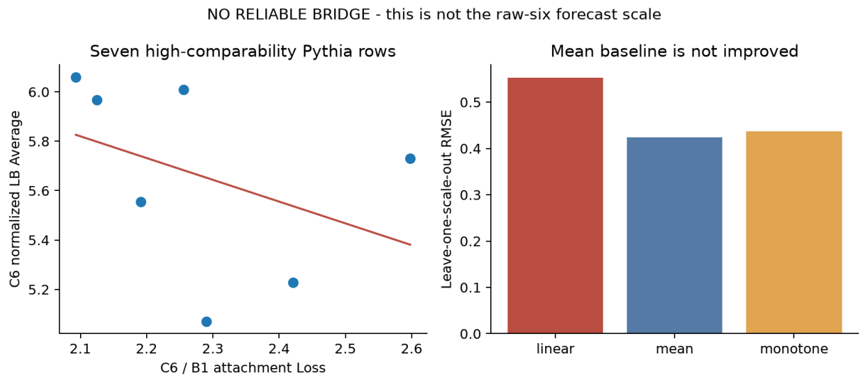
图 12 Loss 与能力桥接的失败诊断。高可比组的留一规模误差未优于均值基准，不能将 Loss 转成榜单能力。
