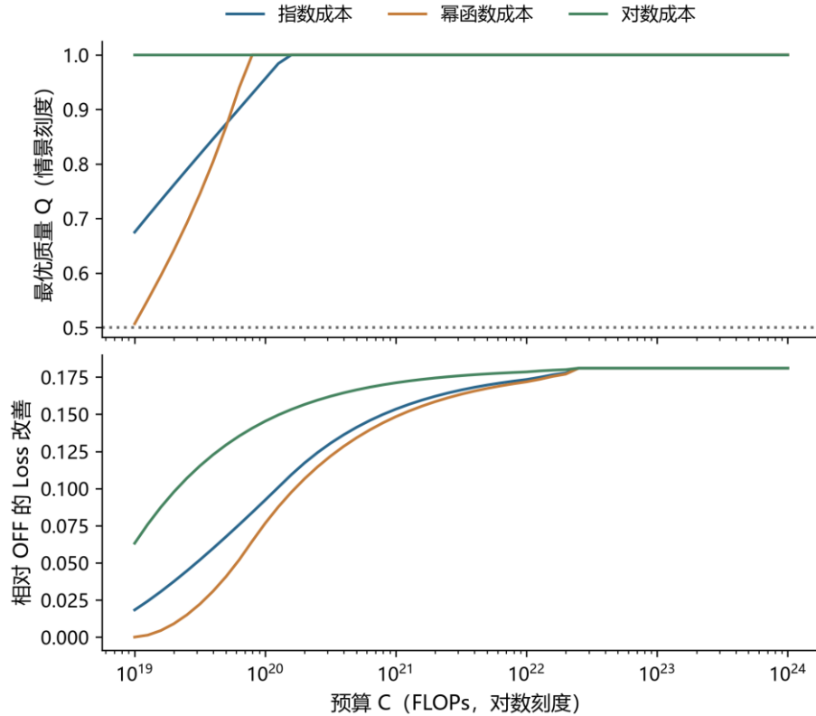
图 6 不同质量成本下的条件配置路径。收益假设来自半合成质量校准，曲线不是实测投资回报。
