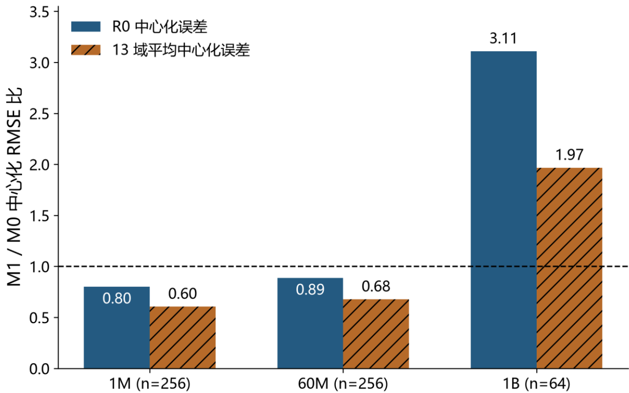
图 10 跨规模配比迁移的中心化误差比。60M 仅部分保持形状，1B 失败；该图不评价绝对 Loss。
