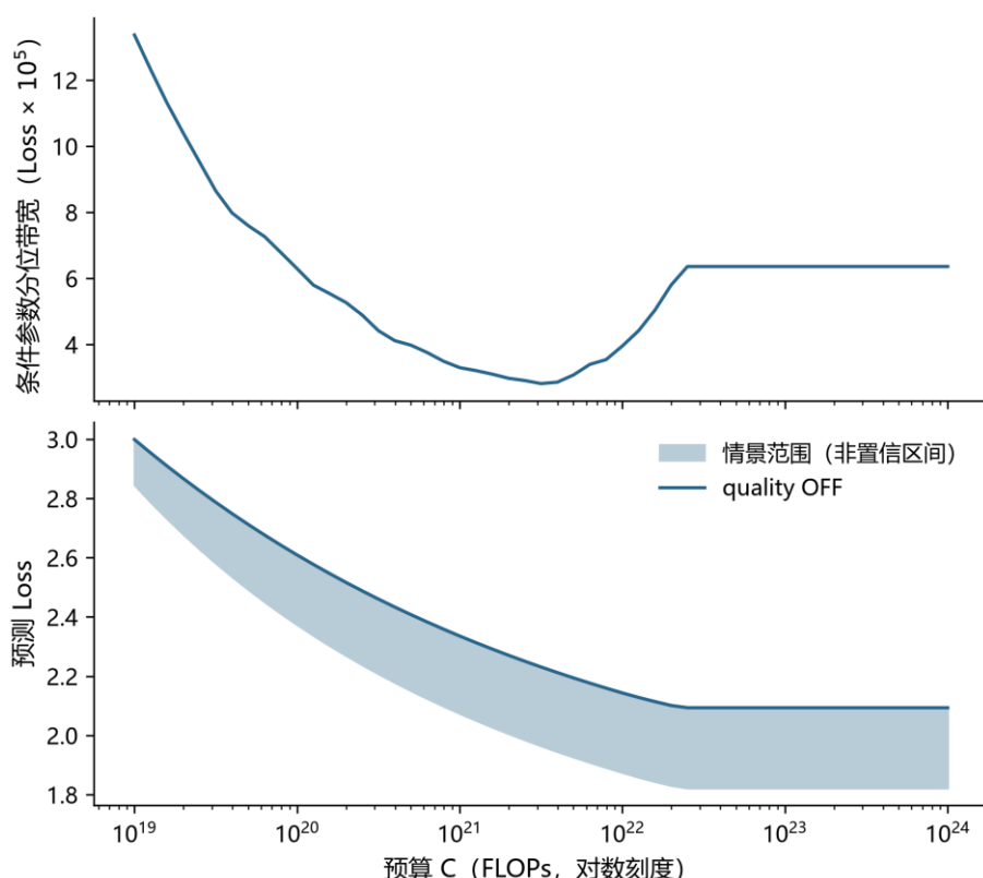
图 7 联合参数传播与机制情景范围。参数条件分位和情景包络分别解释，不把两者合称 95%置信区间。
