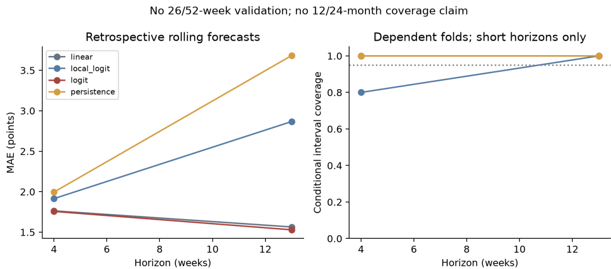
图 13 能力前沿四种动态模型的回溯滚动比较。只存在 4 周和 13 周的可用验证折，长期覆盖仍未知。
