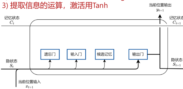
图 3.21: 单个门控神经元主要部件和并行隐藏状态示意图
