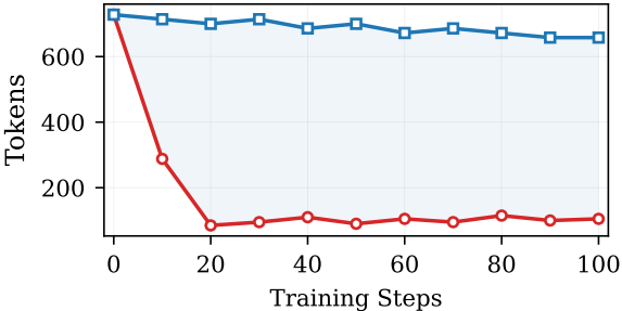
Epistemic Tokens per Response
