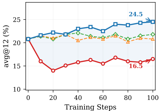
AIME 2025
