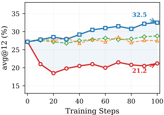
AIME 2024
