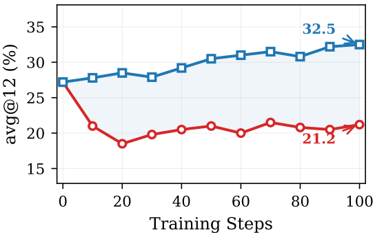
AIME 2024
