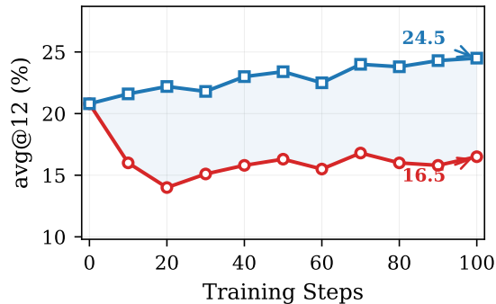
AIME 2025
