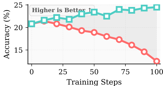
AIME 2025 Accuracy
