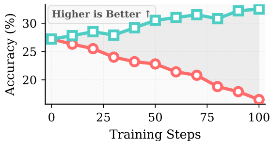
AIME 2024 Accuracy
