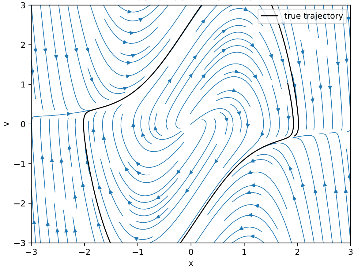
True Van der Pol flow field
