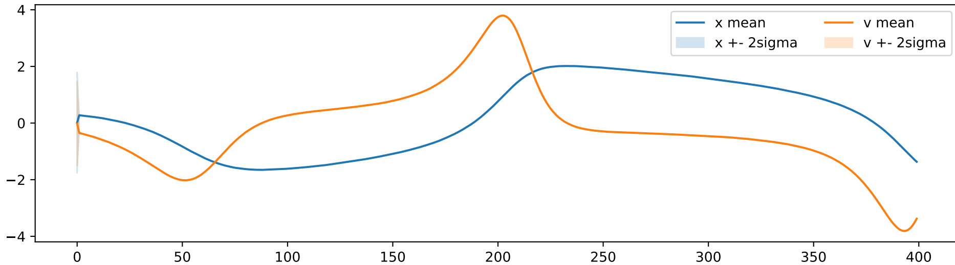
Posterior uncertainty (approx; DiagMVN)
