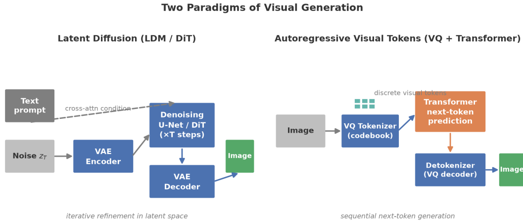
图 1 扩散 vs 自回归：两条生成范式的对比
