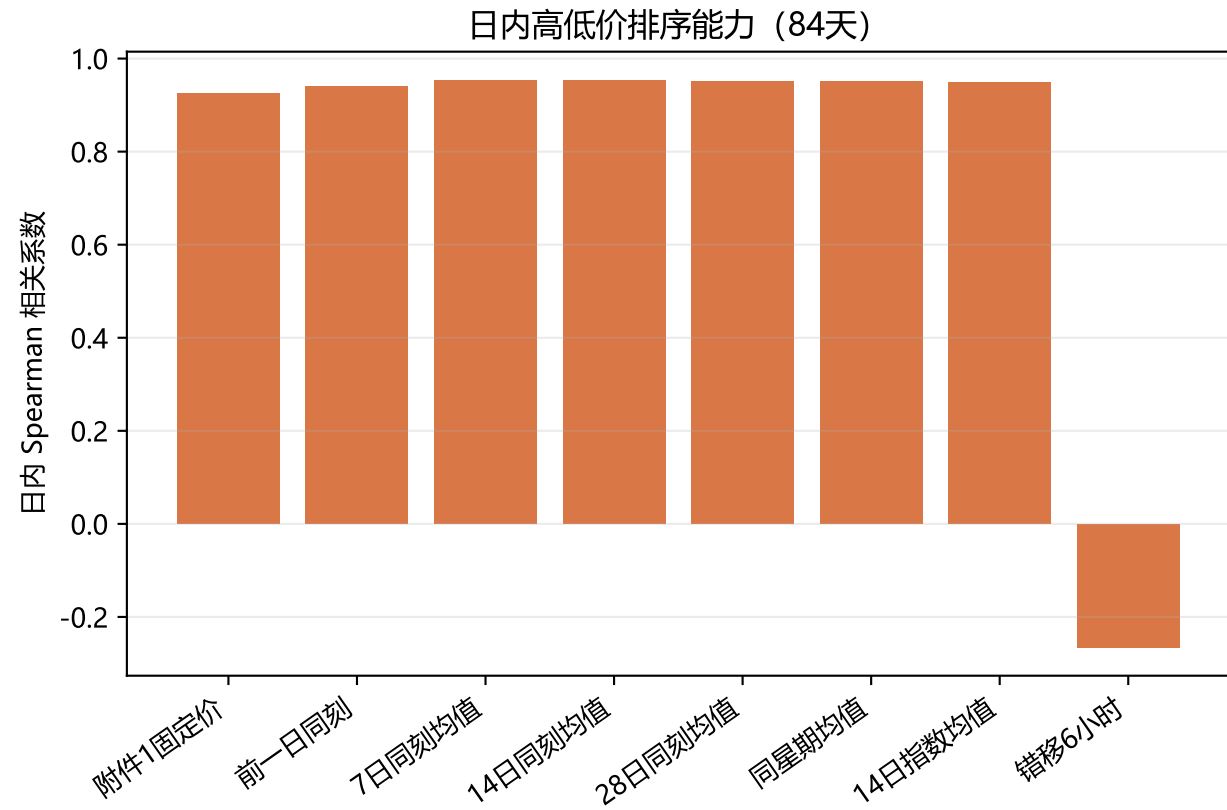
图1 价格预测方法的数值精度与日内排序能力
