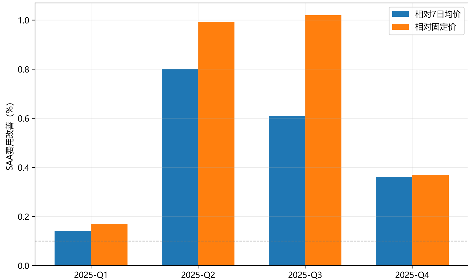
图2 SAA季度稳定性
