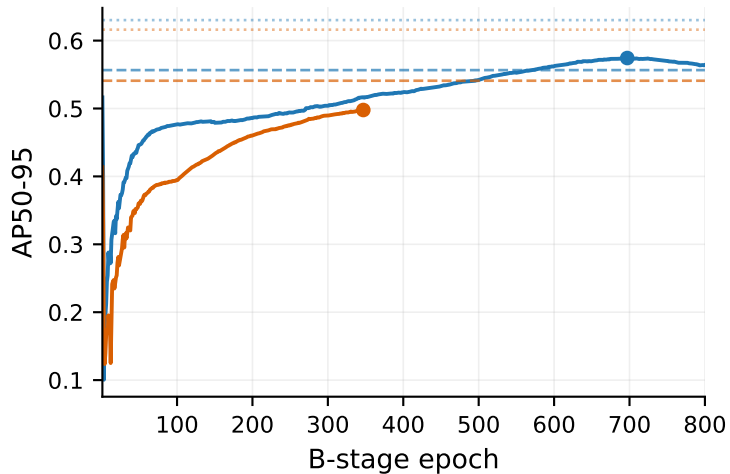
YOLO11n
