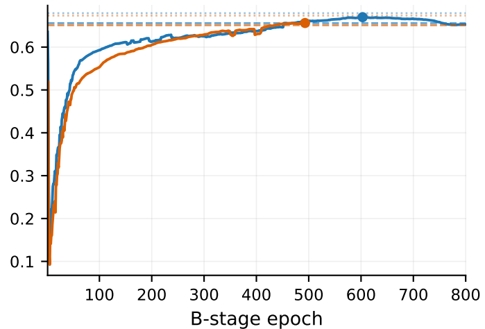
YOLO11m
