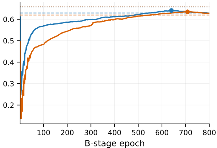
YOLO11s
