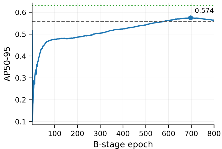
YOLO11n
