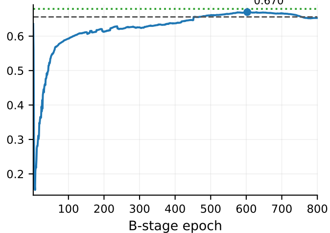
YOLO11m
