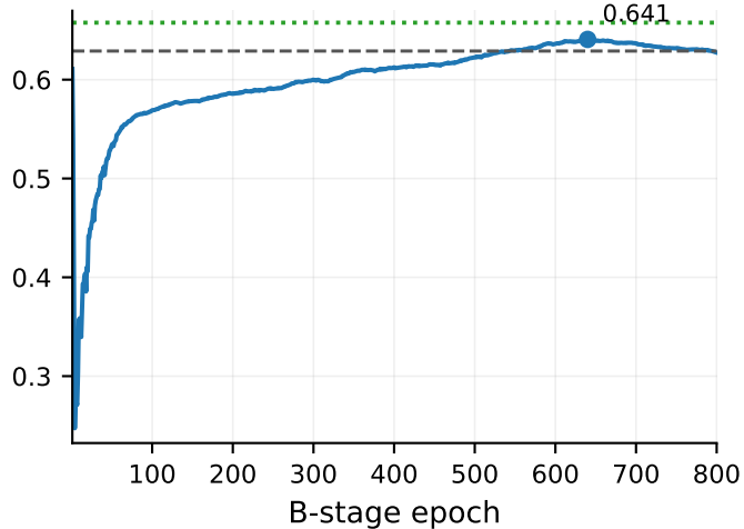
YOLO11s
