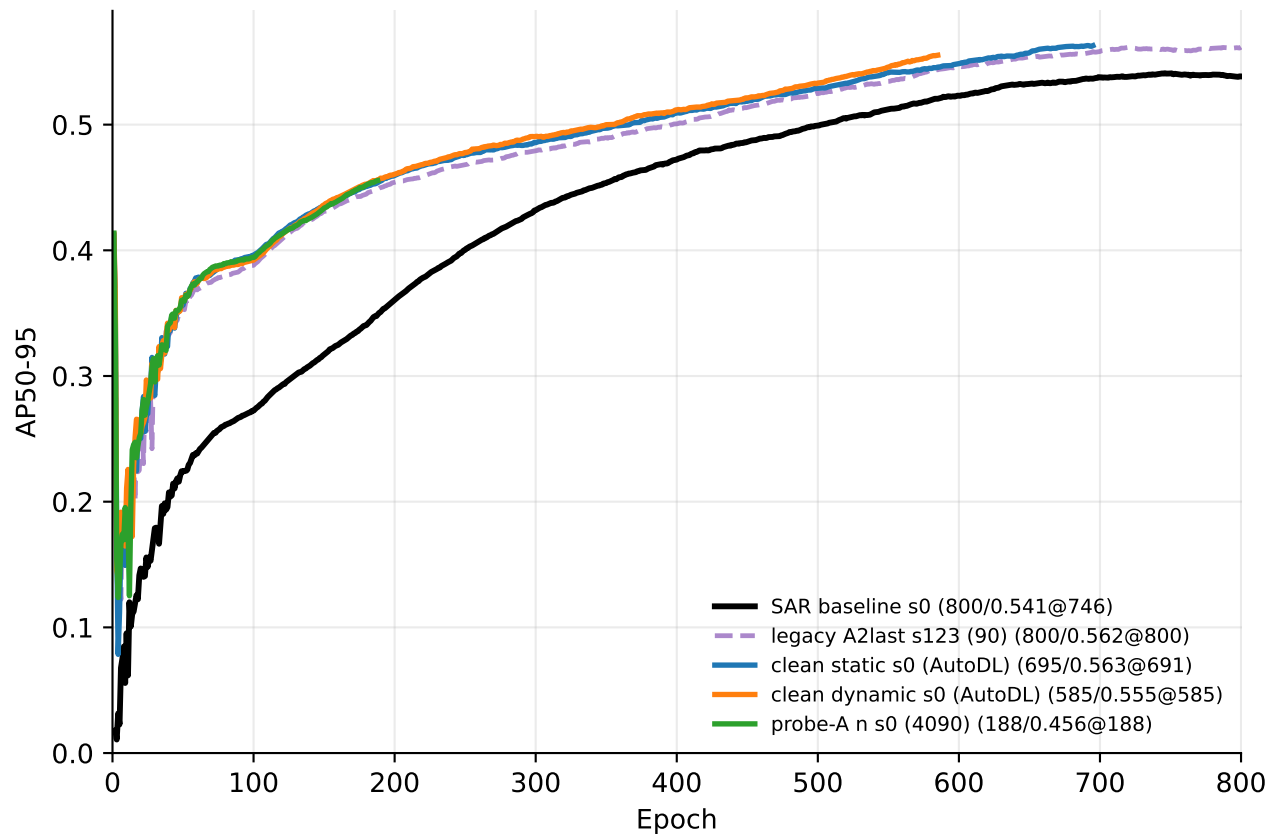
YOLO11n: AP50-95
