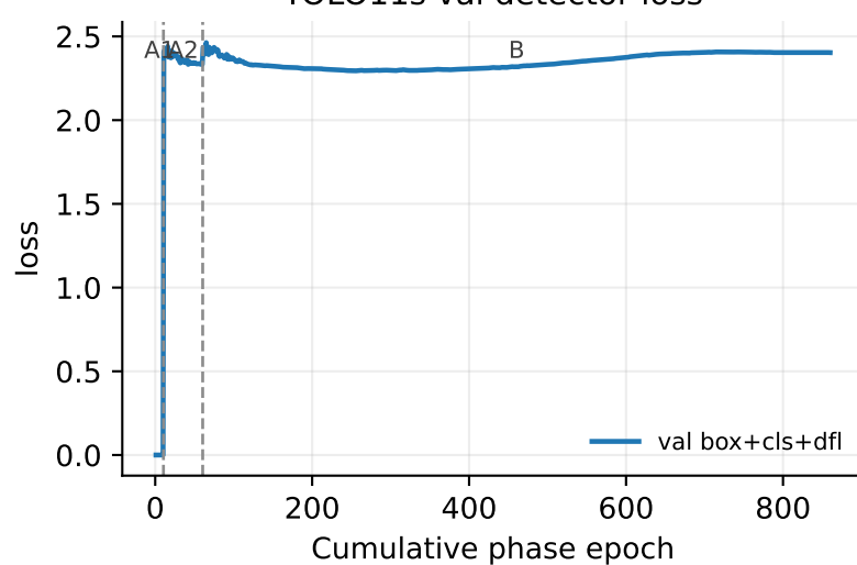
YOLO11s val detector loss
