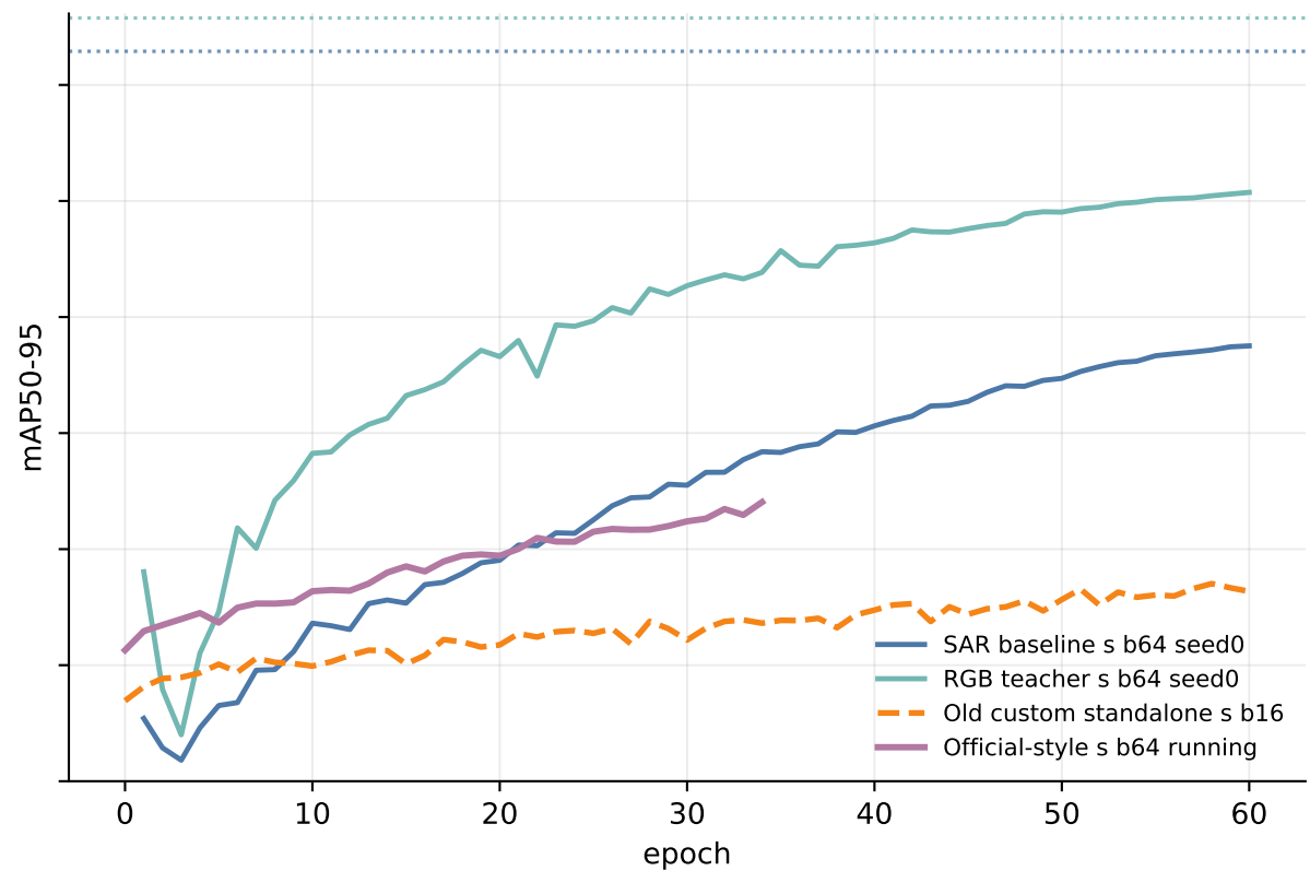
YOLO11s
