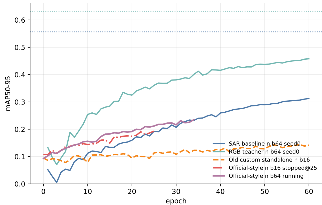
YOLO11n
