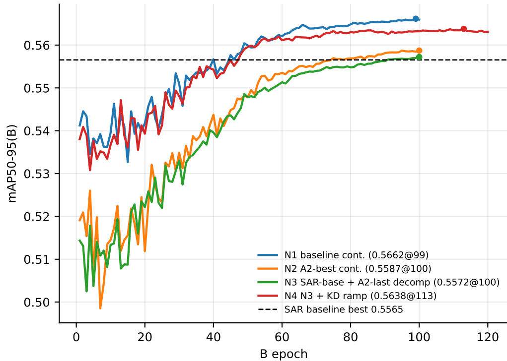
YOLO11n: B-entrance AP curves
