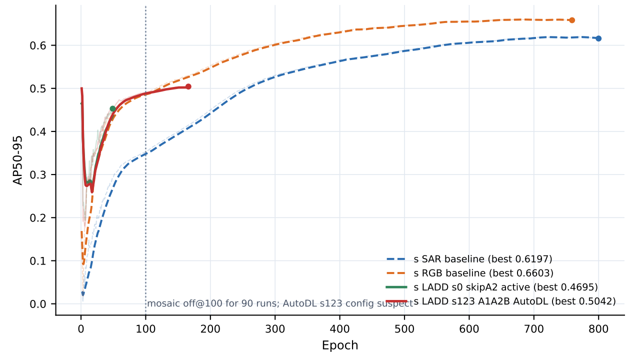
AutoDL YOLO11n nomosaic yolo-init A1 -&gt; B_A2core
