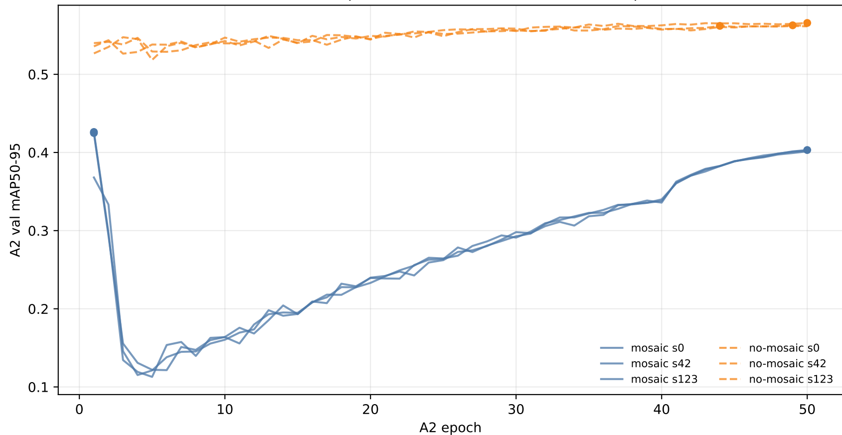
YOLO11n cap2 A2 mAP curves: B loads A2 best.pt
