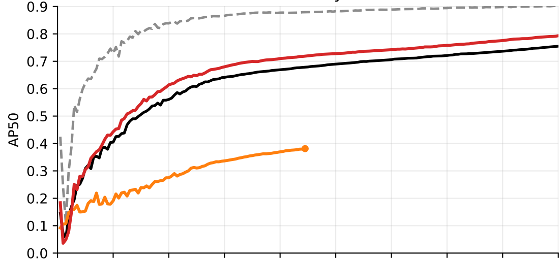
YOLO11m early AP50
