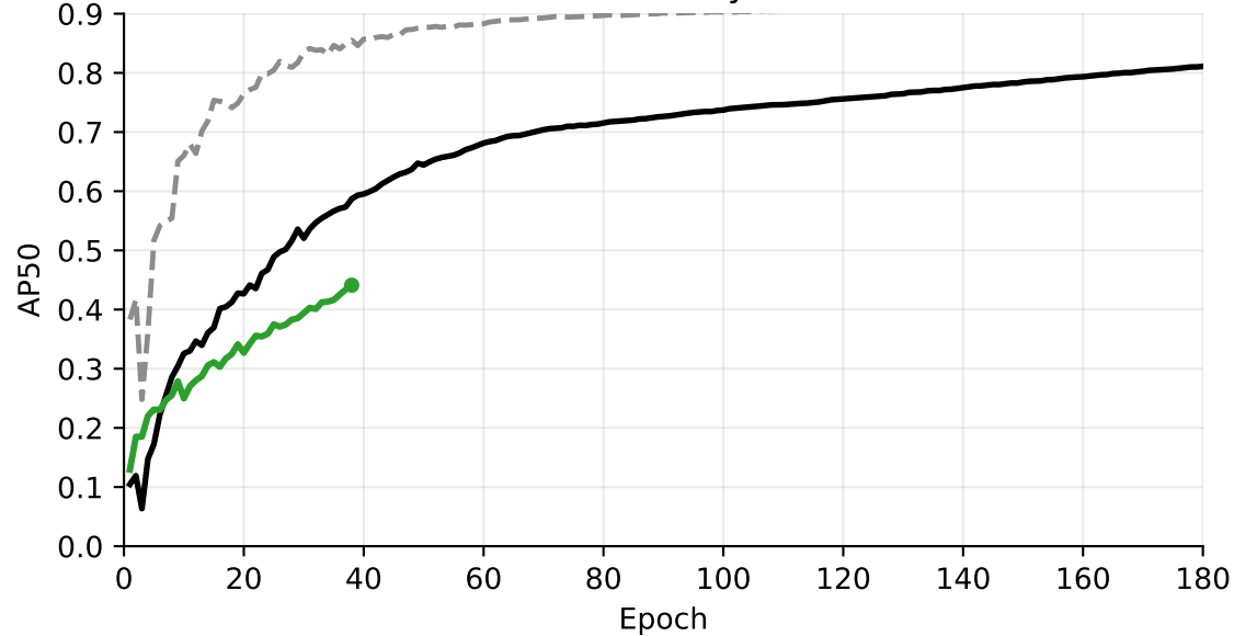
YOLO11m early AP50
