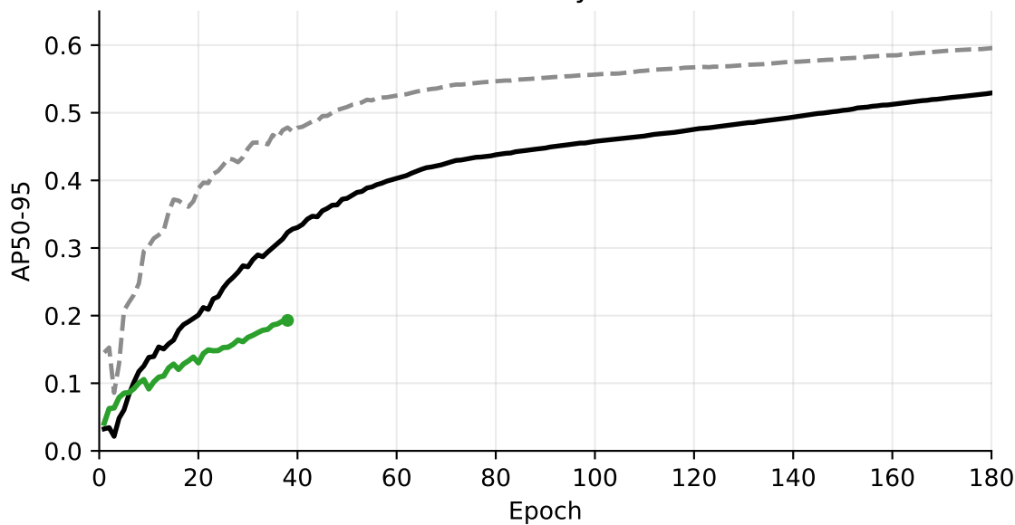
YOLO11m early AP50-95
