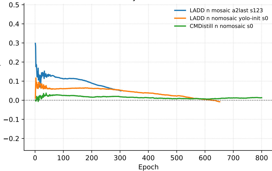
yolo11n
