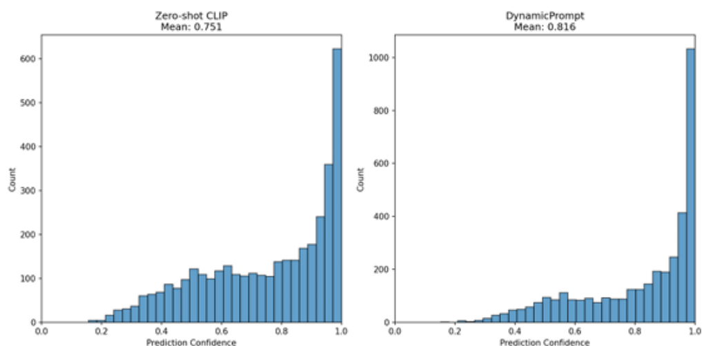
图 4.5 Zero-Shot CLIP 与动态提示词模型的预测置信度分布
