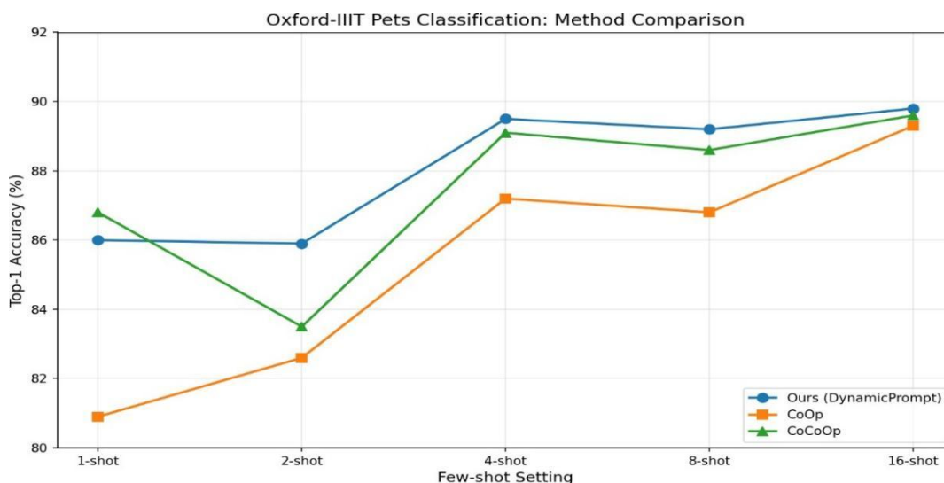
图 4.2 不同方法准确率随 Shot 数变化的趋势
