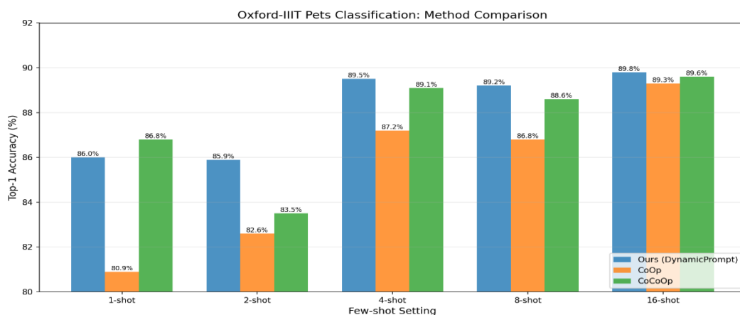
图 4.1 不同方法在各 Shot 设置下的准确率对比
