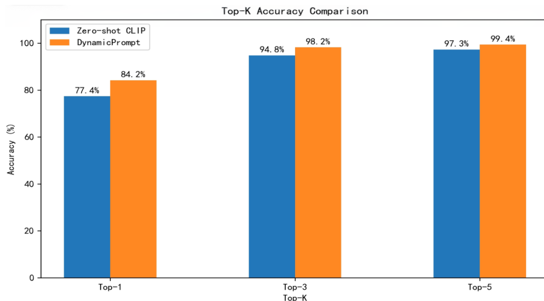
图 4.4 Zero-Shot CLIP 与动态提示词模型的 Top-k 准确率对比
