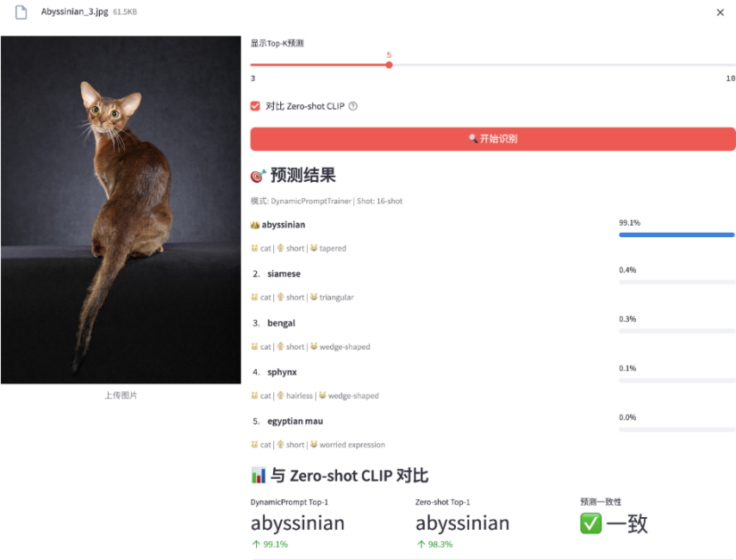
图 5.3 动态提示词模型与原始 CLIP 的对比结果
