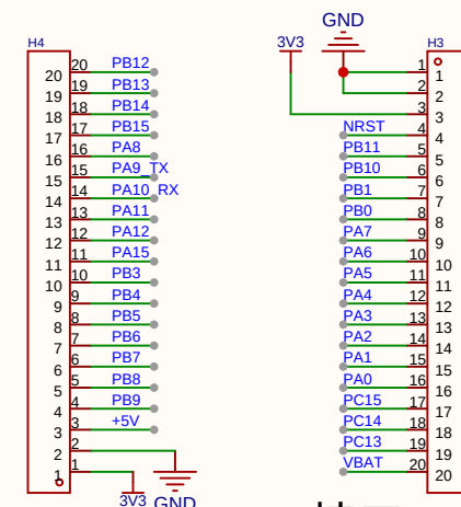
IO接口
