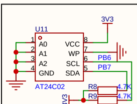
EEPROM
