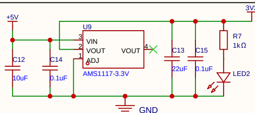
3V3降压电路
