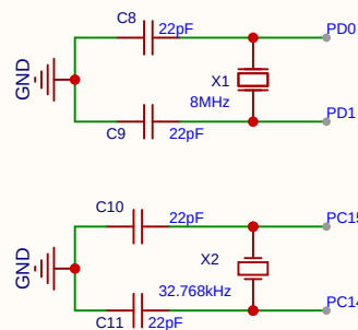
晶振电路
