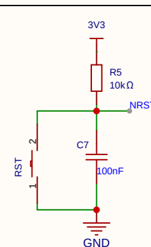
复位电路
