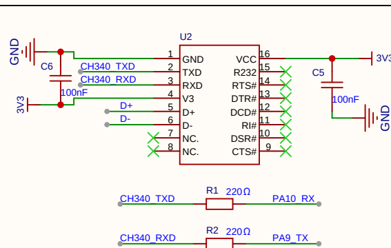
CH340
