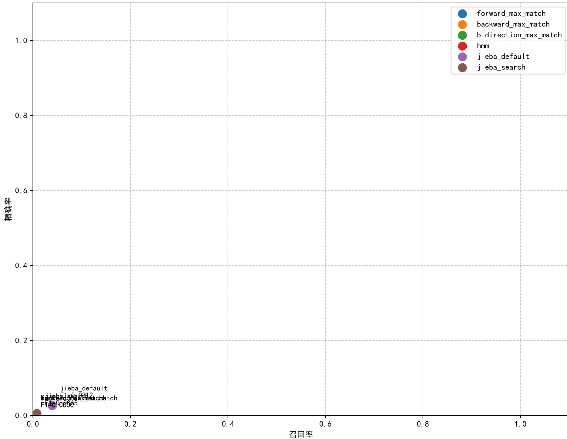
各分词方法的精确率-召回率
