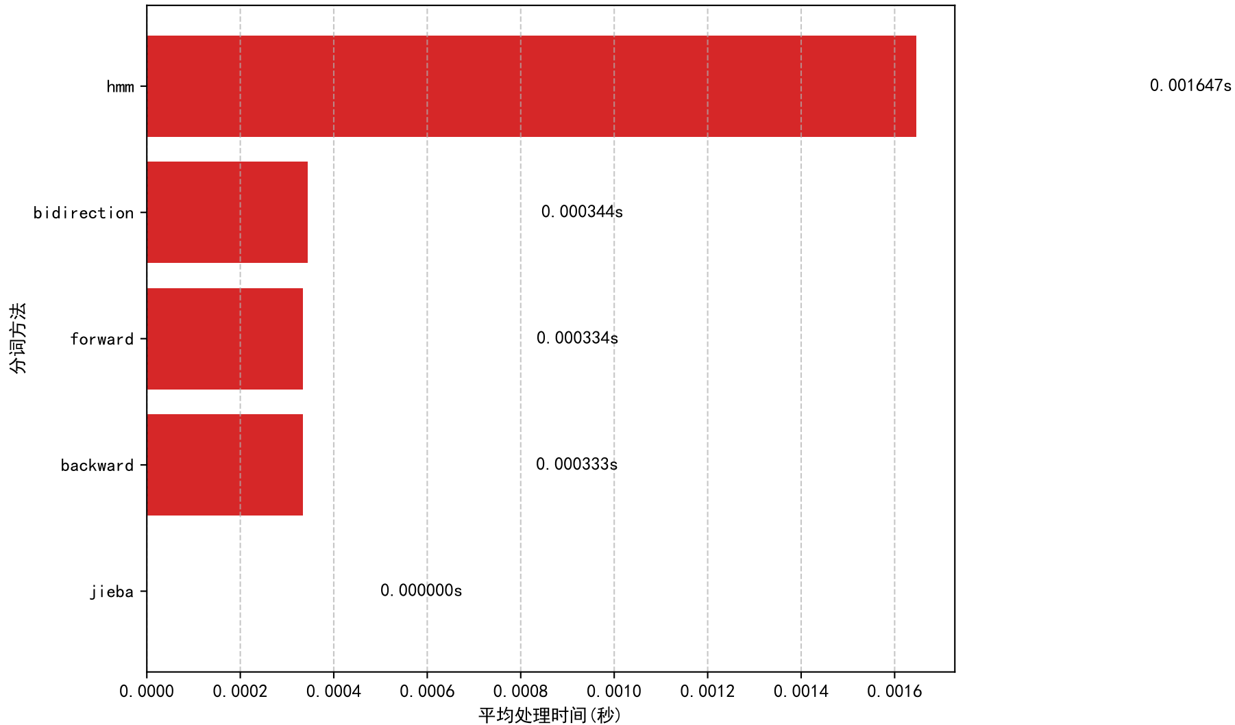
各分词方法速度对比
