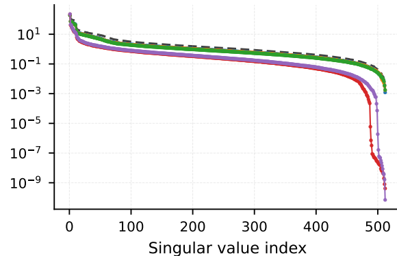
Layer 19 (linear)
