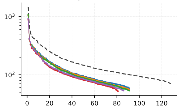
Layer 3 (conv2)
