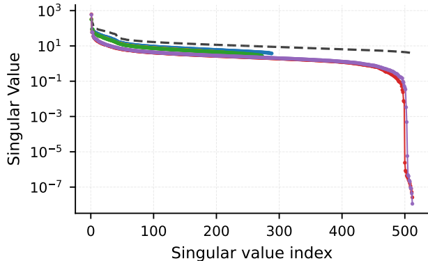
Layer 14 (conv5)
