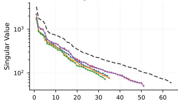
Layer 0 (conv1)
