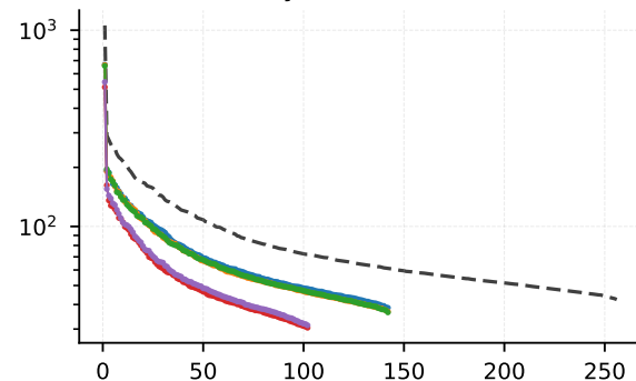
Layer 7 (conv3)
