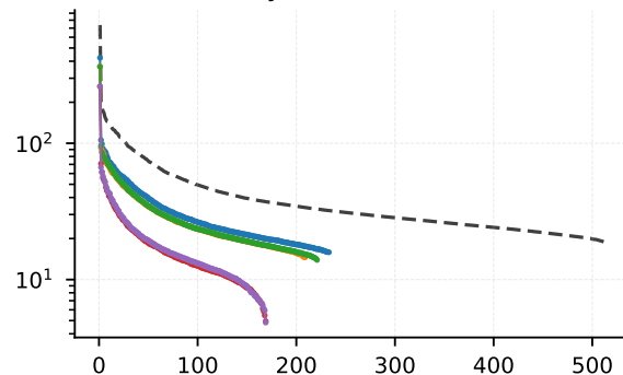
Layer 11 (conv4)
