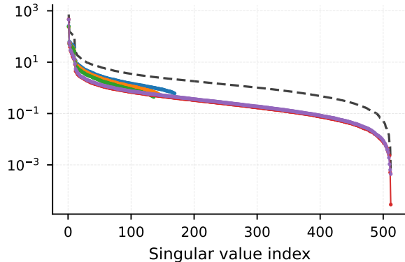
Layer 16 (conv5)
