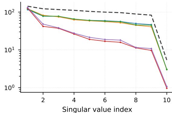
Layer 21 (last layer)
