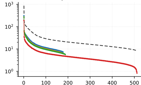
Layer 12 (conv4)
