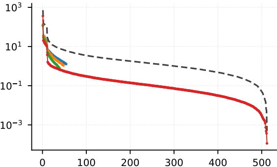
Layer 16 (conv5)
