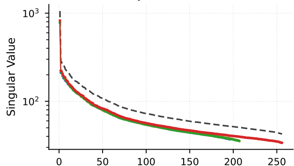
Layer 7 (conv3)
