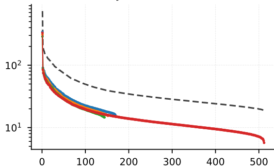
Layer 11 (conv4)
