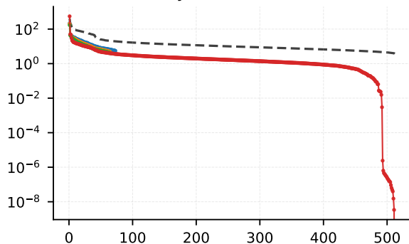
Layer 14 (conv5)
