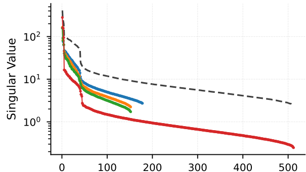
Layer 15 (conv5)
