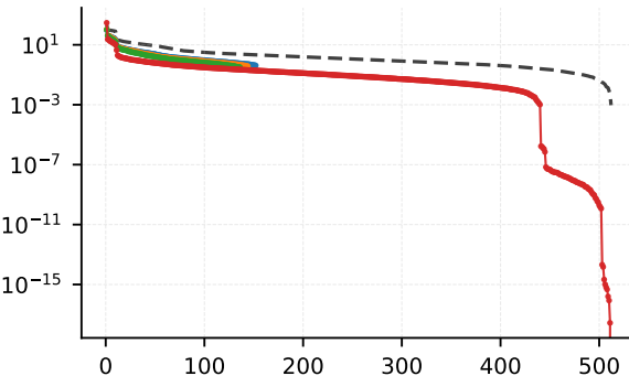
Layer 19 (linear)
