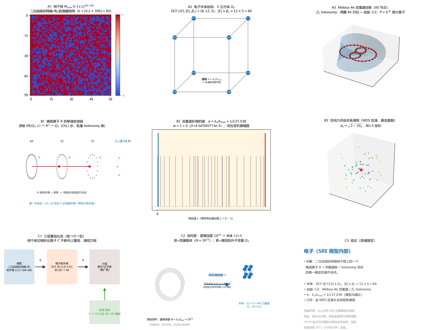
图 10-1: 相干核、本体 Q_3 、Möbius 双覆盖、稀疏算子收敛、 \alpha 谱、三层 RG 与逻辑深度折叠的整体示意（模型内部图景，非现实测量）。矢量版见 figures/sre_electron_schematic.svg。
