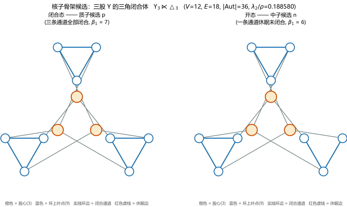
图 1：左为闭合态（质子候选，三条环边全部闭合），右为开态（中子候选，一条环边休眠未闭合，红色虚线）。橙色为股心（3 个），蓝色为环上叶点（9 个），蓝色实线为闭合通道。开态与闭态的唯一差别是"少一个闭合单元"（三角环数 3 \rightarrow 2 ），这正是第 6.3 节破缺量级论证的结构基础。
