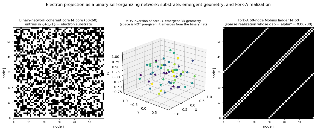
图 9-1：电子 60 投影作为二元网络相干核的涌现子结构（模型内部图景，非现实测量）。
