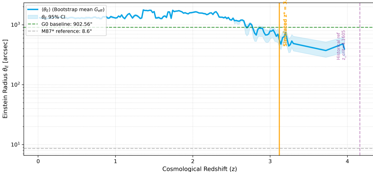
图4 引力透镜爱因斯坦半径随红移演化。蓝色实线为Bootstrap系综平均结果，浅蓝色阴影为95%置信区间；绿色虚线为 G_0 基准爱因斯坦半径；橙色实线标记仿真相变 z^* = 3.13 ，紫色虚线为历史参考 z_{\text{crit}} = 4.1605 。
