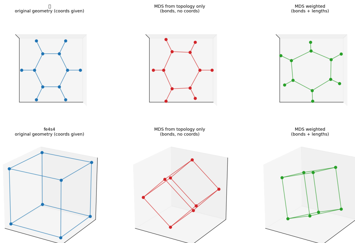
图 12-1: 电子关系矩阵的 MDS 三维反演嵌入 (模型内部关系嵌入, 非现实三维位置测量)。
