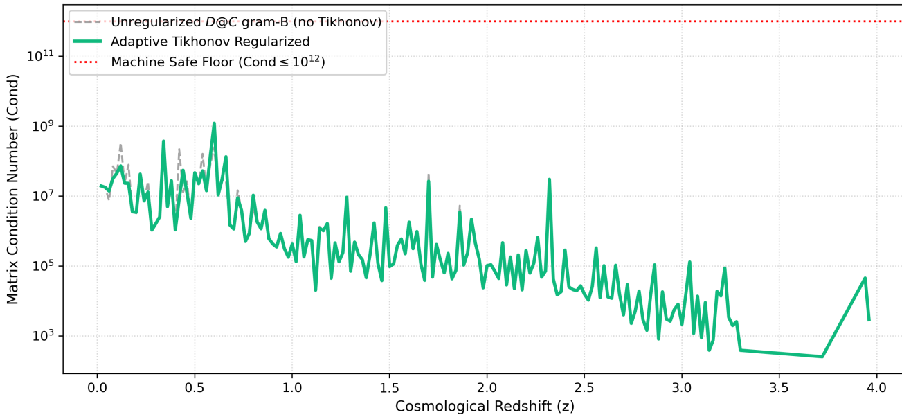
图 3 随宇宙学红移 z 变化的矩阵条件数数值稳定性诊断。灰色虚线：未正则化度量矩阵；绿色实线：采用自适应吉洪诺夫流形正则化后的结果，条件数被约束在数值稳定区间；红色水平线代表机器安全条件数上限 \text{Cond} \leq 10^{12} 。
