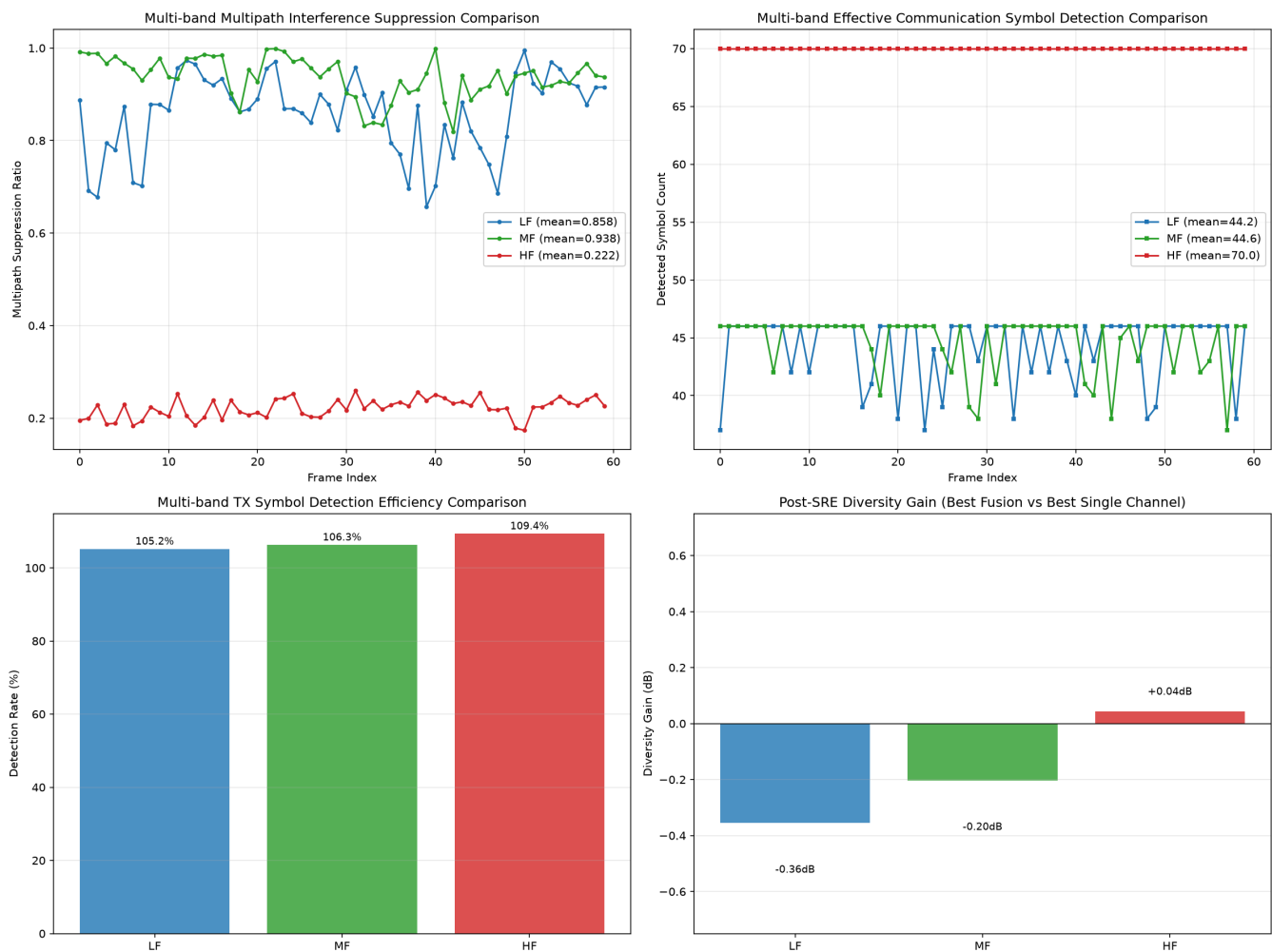
图1 多频段水声通信SRE处理综合性能对比。左上：多径干扰抑制比时序；右上：有效通信符号检出计数时序；左下：发射符号检测效率；右下：SRE处理后分集增益（融合输出对比最优单通道）。
