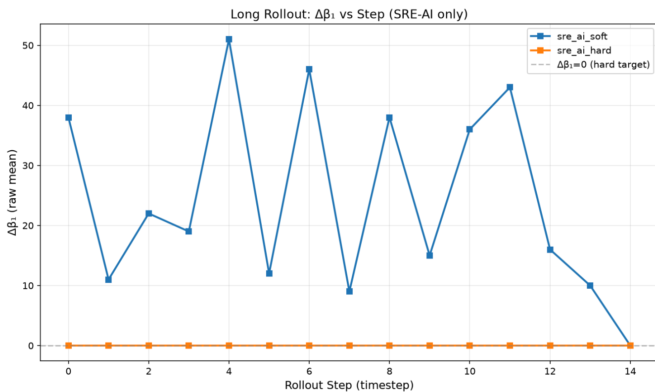
图3(b): 滚动步- \Delta\beta_1 (仅SRE-AI, 基线无该指标不参与对比)
