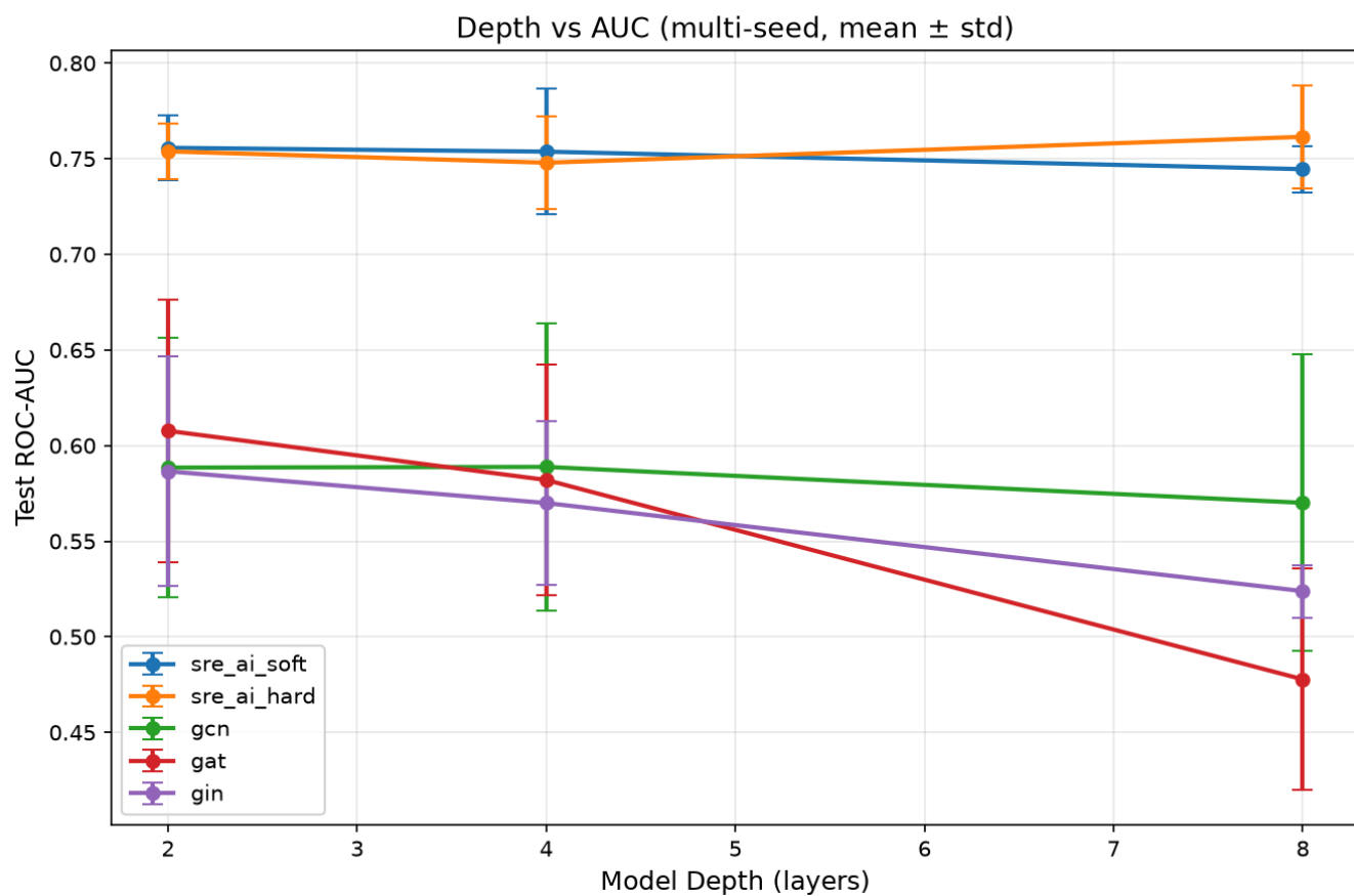
图1：层数-AUC曲线（多种子带误差棒，3种子）
