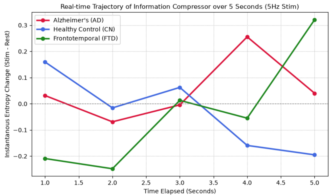
图1 5秒内信息压缩器实时轨迹（5Hz刺激）。纵轴：瞬时熵变化(刺激-静息)；横轴：经过时间(秒)。红色：阿尔茨海默AD组；蓝色：健康对照CN组；绿色：额颞叶痴呆FTD组。
