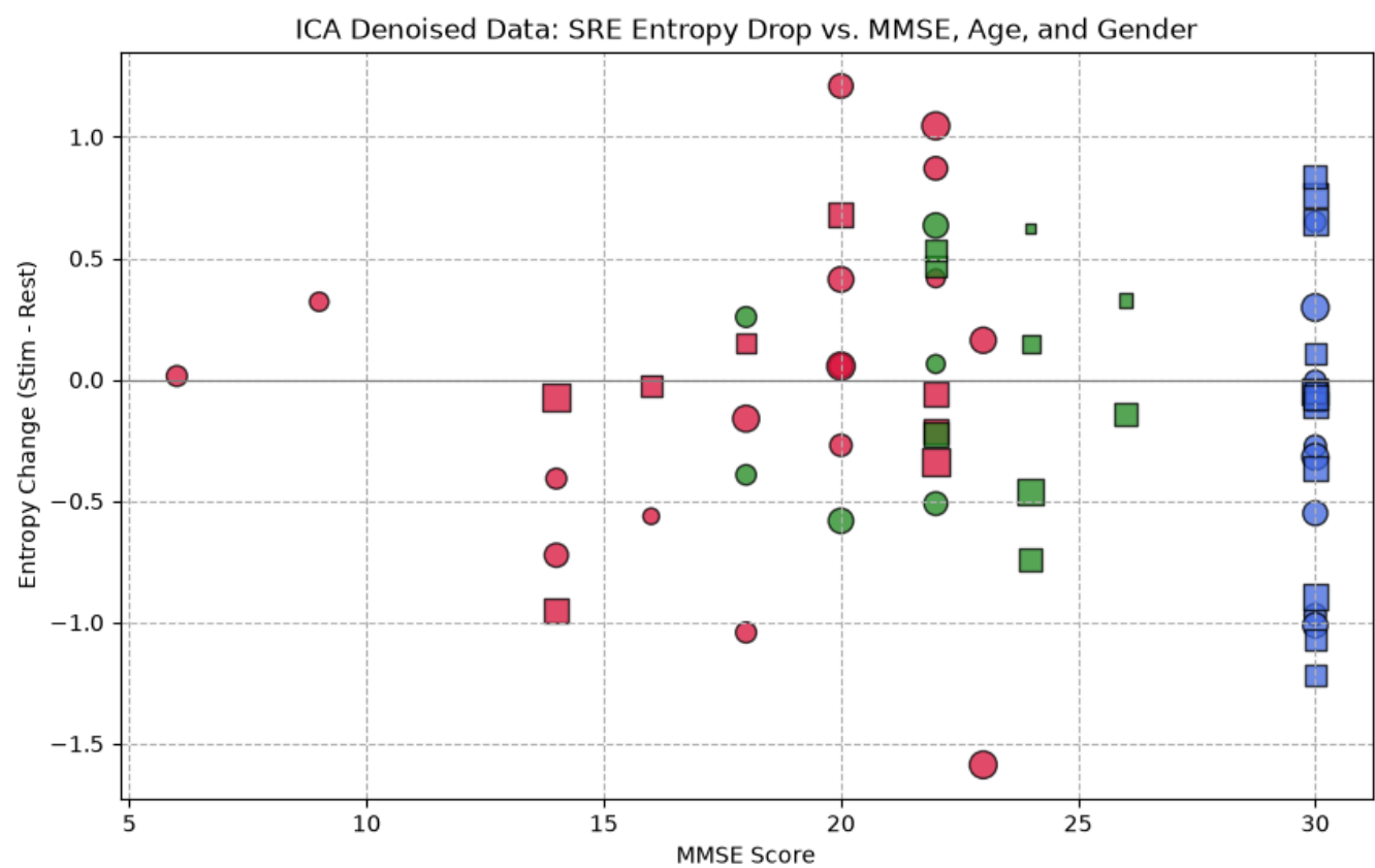
图2 ICA降噪数据：SRE熵下降对比MMSE评分、年龄与性别。横轴MMSE量表得分，纵轴瞬时熵变化(刺激-静息)。
