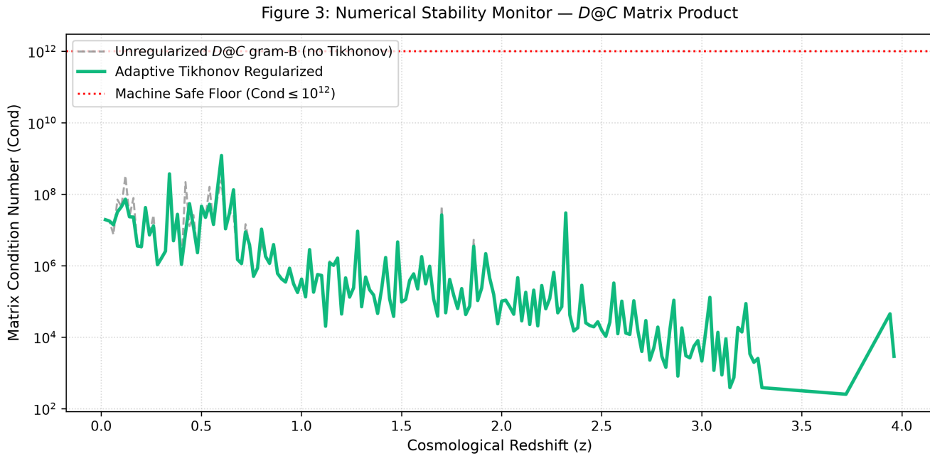
图 3 随宇宙学红移 z 变化的矩阵条件数数值稳定性诊断。灰色虚线：未正则化度量矩阵；绿色实线：采用自适应吉洪诺夫流形正则化后的结果，条件数被约束在数值稳定区间；红色水平点线代表机器安全条件数上限 \text{Cond} \leq 10^{12} 。
