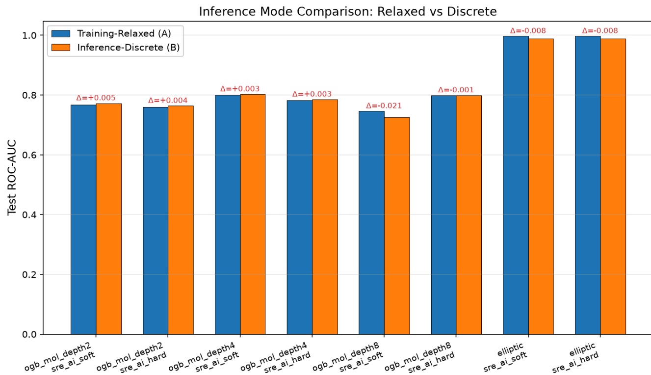
图5：松弛推理(A)与原生离散推理(B)AUC对比柱状图，柱上方标注 \Delta AUC差值
