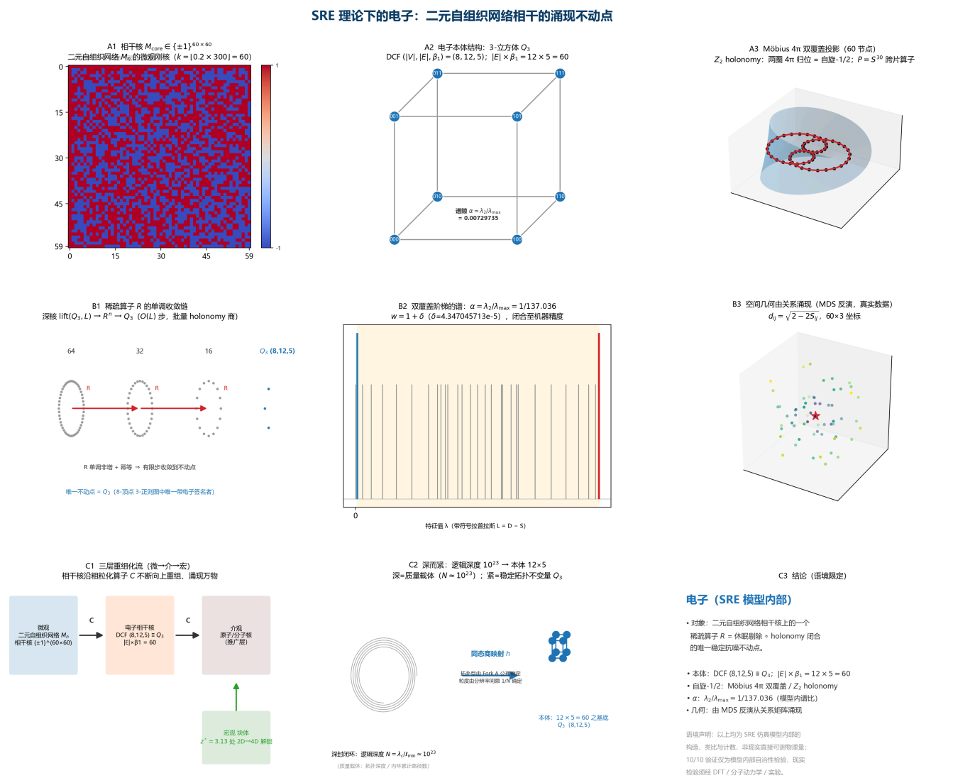
图 10-1 (figures/sre_electron_schematic.png)：SRE 框架下电子的综合示意图（3×3 面板）：A 行为相干核热图 / Q_3 本体 / Möbius 4\pi 双覆盖；B 行为稀疏算子 R 的收敛（ 64 \rightarrow 8 ）、 \alpha 谱（真实 w=1+\delta ）与 MDS 三维反演；C 行为三层 RG 流、 10^{23} \rightarrow 12 \times 5 逻辑深度折叠与结论声明。
