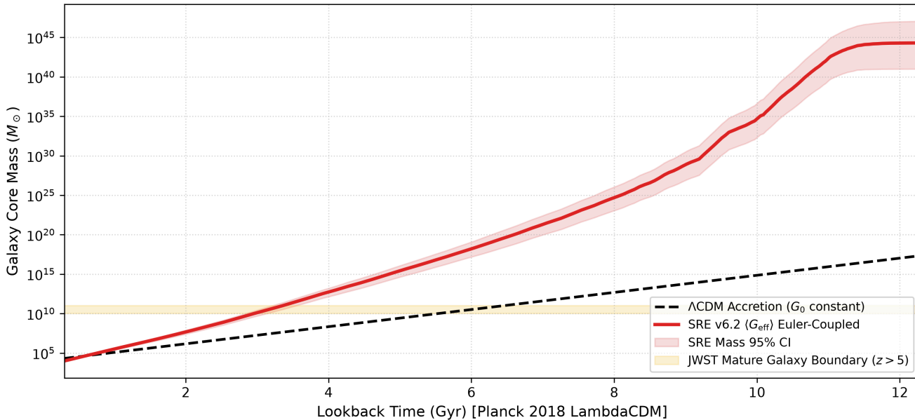
图 2 原初因果核质量累积对比。黑色虚线：标准 \Lambda -CDM 模型，引力常数取静态 G_0 下的质量增长曲线；红色实线：高维解锁相中动态 \langle G_{\text{eff}} \rangle 作用下 SRE 增强吸积模型；浅黄色阴影带标记 JWST 观测得到的 z > 5 成熟星系的质量边界。横轴为宇宙回溯时间，单位为吉年（Gyr）；粉色阴影为Bootstrap仿真95%质量置信区间。SRE冷却增强效应能够在宇宙允许的时标内达到观测的星系核质量。
