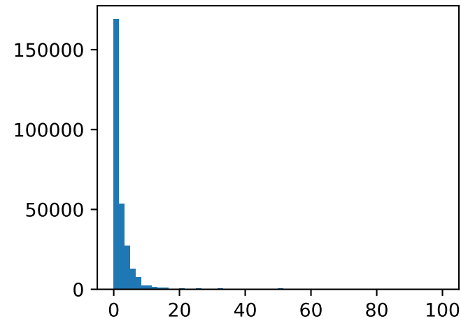
% mitochondrial
